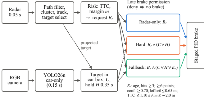
Hình 1. Chuỗi xử lý dừng chung từ cảm biến đến phanh. Mọi chính sách nhận cùng một yêu cầu phanh radar B_r và cùng xác nhận chỉ-ô-tô C /giữ xác nhận H , và chỉ khác nhau ở bước cấp quyền ở khâu cuối: cổng cứng từ chối B_r khi không có hộp ô tô tại mục tiêu được chiếu; dự phòng còn cấp quyền cho B_r khi điều kiện khẩn cấp E_r thỏa mãn.
