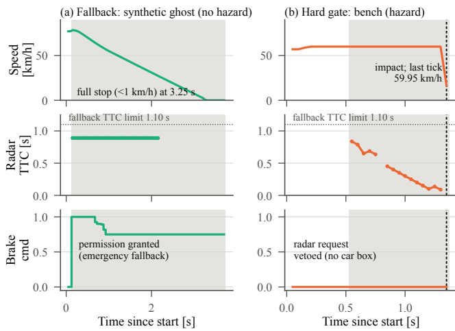
Hình 2. Nhặt ký theo tick đã đóng băng. (a) Dự phòng, bóng ma tổng hợp sáu điểm: cấp quyền khẩn cấp tại 0.15 s và dừng hẳn. (b) Cổng cứng, ghế băng trong tập giữ lại: yêu cầu của radar bị phủ quyết cho đến lúc va chạm (nét đứt). Màu xám: có yêu cầu radar B_r . Cách chọn: lượt chạy có các đại lượng mô tả mức độ nghiêm trọng bằng trung vị của chính sách (tốc độ bắt đầu phanh, thời lượng và giảm tốc cực đại của bóng ma trên 20 lượt chạy; tốc độ trước và chạm của ghế băng trên năm lượt chạy), chọn mã kịch bản/lượt chạy nhỏ nhất khi bằng nhau.
