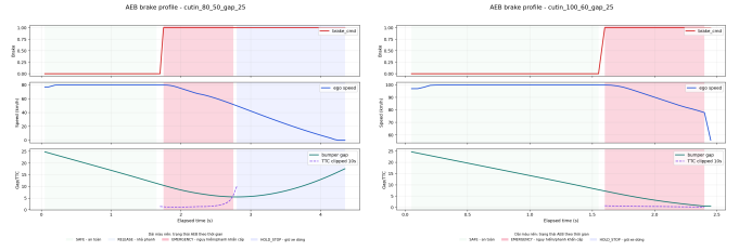
Hình 3. Biểu đồ phanh cut-in: đạt tại 80/50 km/h và không đạt tại 100/60 km/h với gap đầu 25 m.
