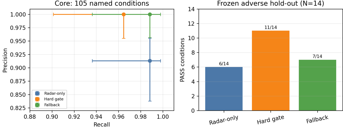
Fig. 1. Kết quả theo từng điều kiện đã khóa. Trái: precision–recall của bộ chính và khoảng Wilson mô tả trên điều kiện định danh được xây dựng. Phải: số điều kiện PASS trên bộ hold-out bất lợi gồm 14 điều kiện. Các bộ này không cho biết tần suất tình huống ngoài đường. Hình giữ nhãn tiếng Anh để đối chiếu với bản nộp.
