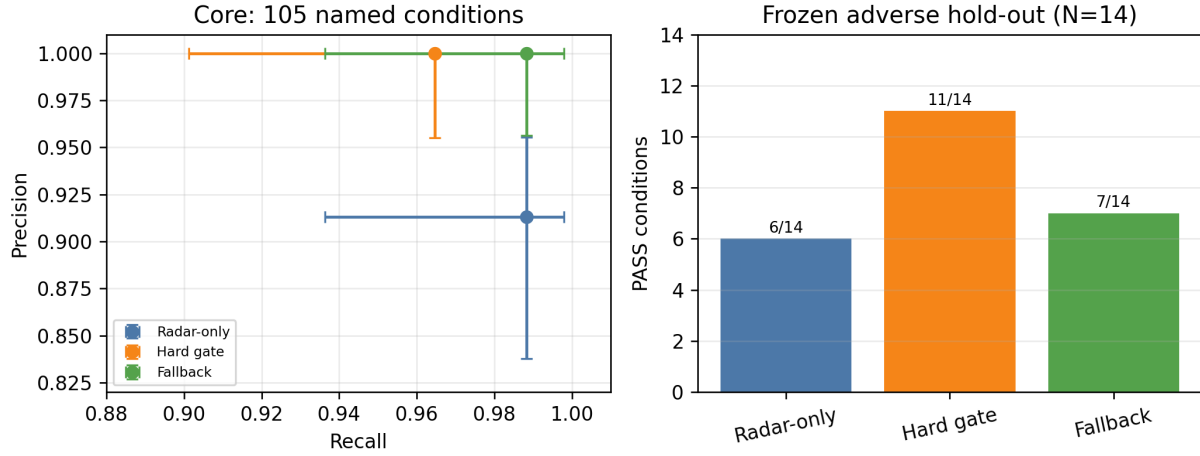
Fig. 1. Kết quả theo từng điều kiện đã khóa. Trái: precision–recall của bộ chính và khoảng Wilson mô tả trên điều kiện định danh được xây dựng. Phải: số điều kiện PASS trên bộ hold-out bất lợi gồm 14 điều kiện. Các bộ này không cho biết tần suất tình huống ngoài đường. Hình giữ nhãn tiếng Anh để đối chiếu với bản nộp.
