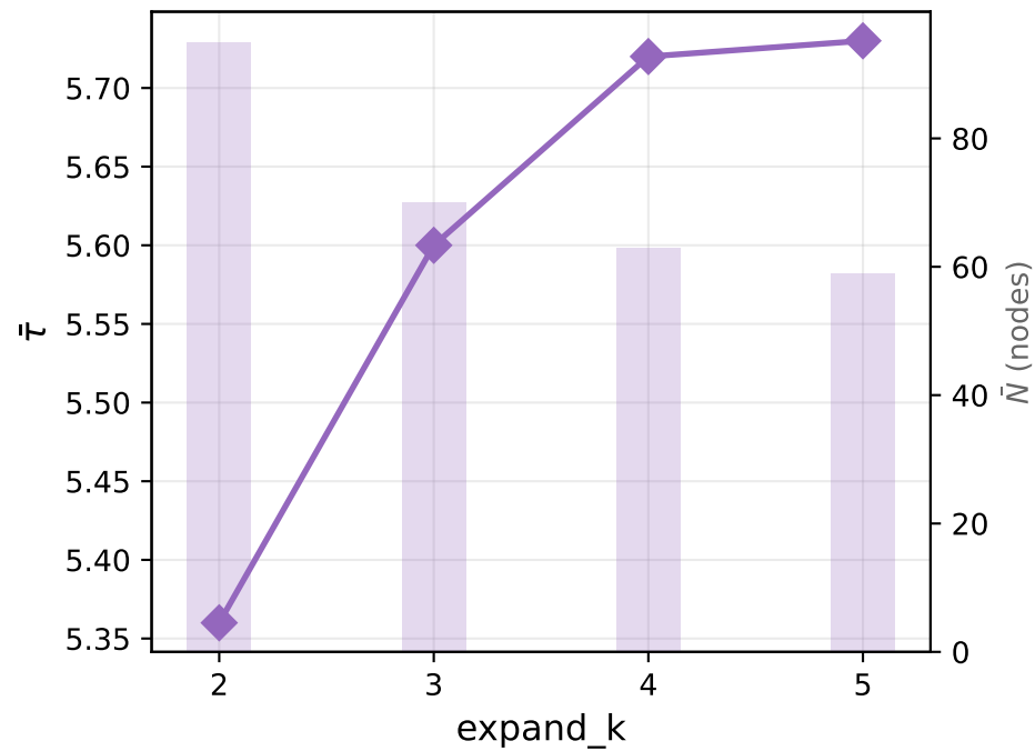
MT-Bench
