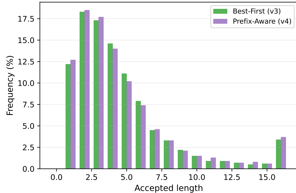
MT-Bench
