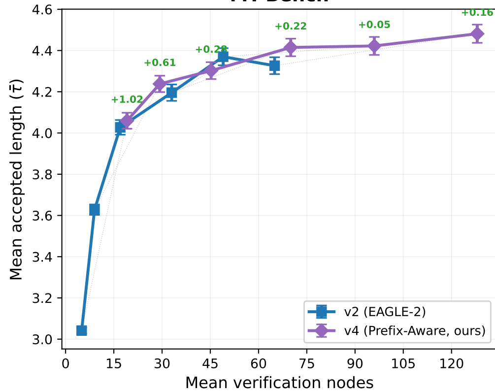
MT-Bench
