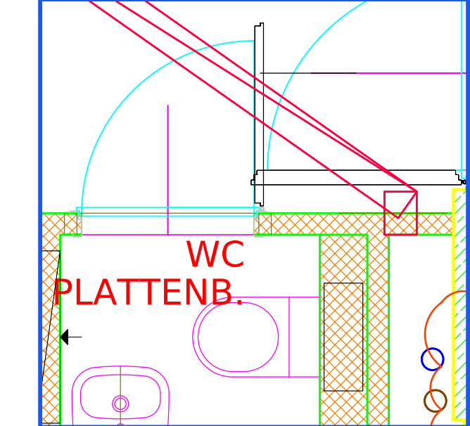
Lücke in der Wand + gerade Linie (Türblatt) + Viertelkreis (Weg der Türkante).
