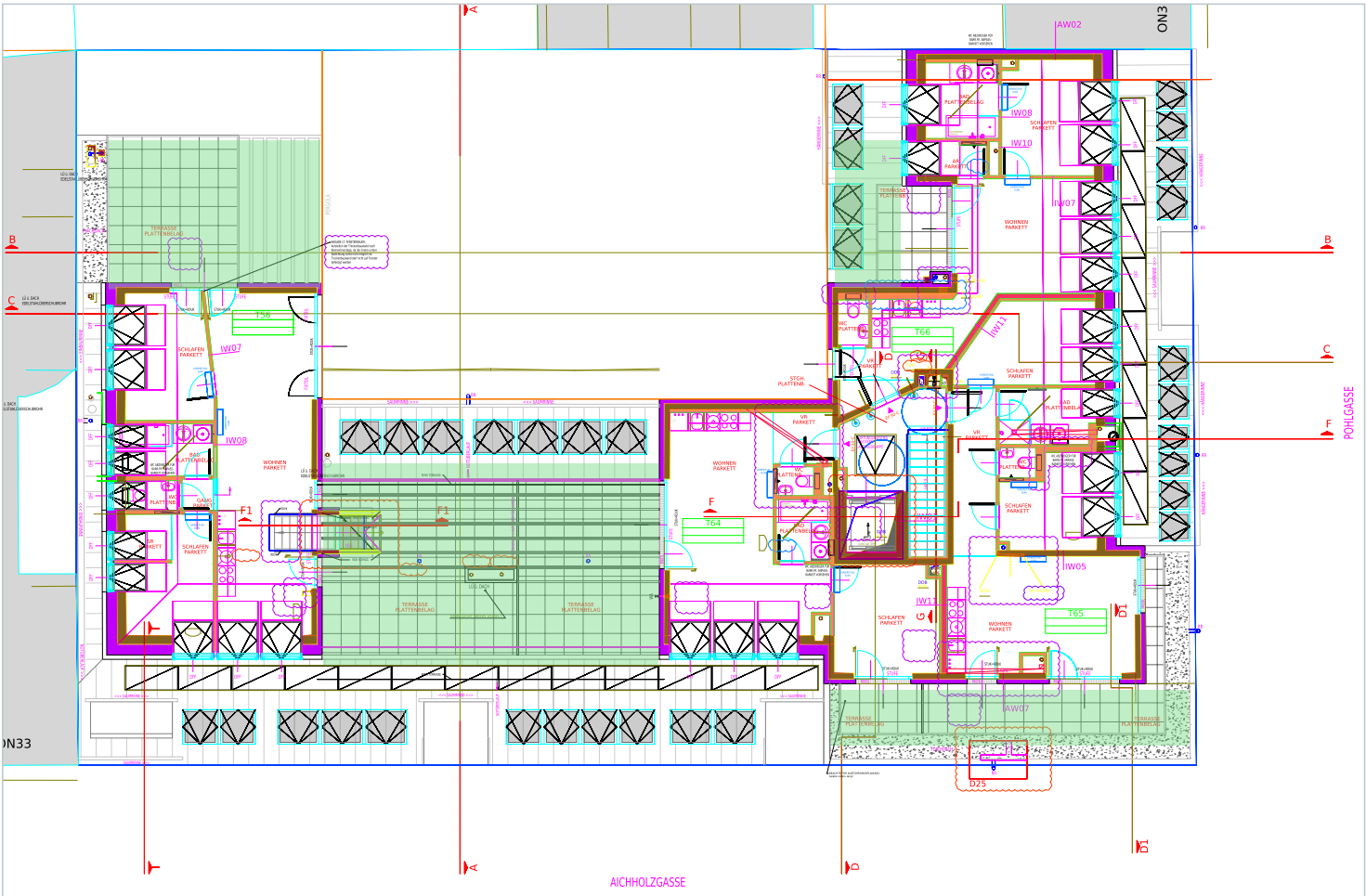
2. Dachgeschoss (Wände rot, Terrassen hellgrün)
