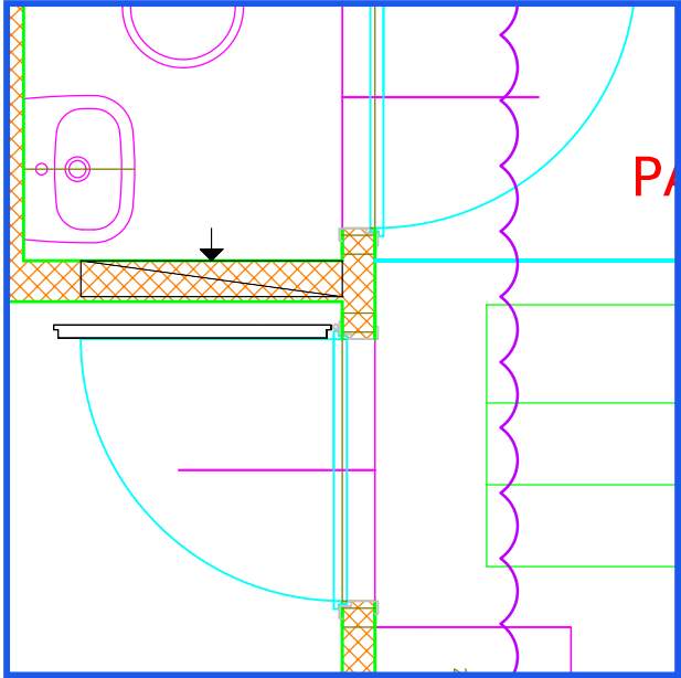
Lücke in der Wand + gerade Linie (Türblatt) + Viertelkreis (Öffnungsweg).
