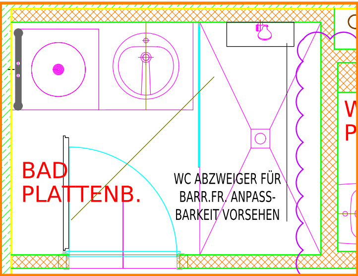
Ovale = WC-Schüssel, runde Formen in Rechtecken = Waschbecken. Dünn gezeichnet, weil sie am Boden stehen.
