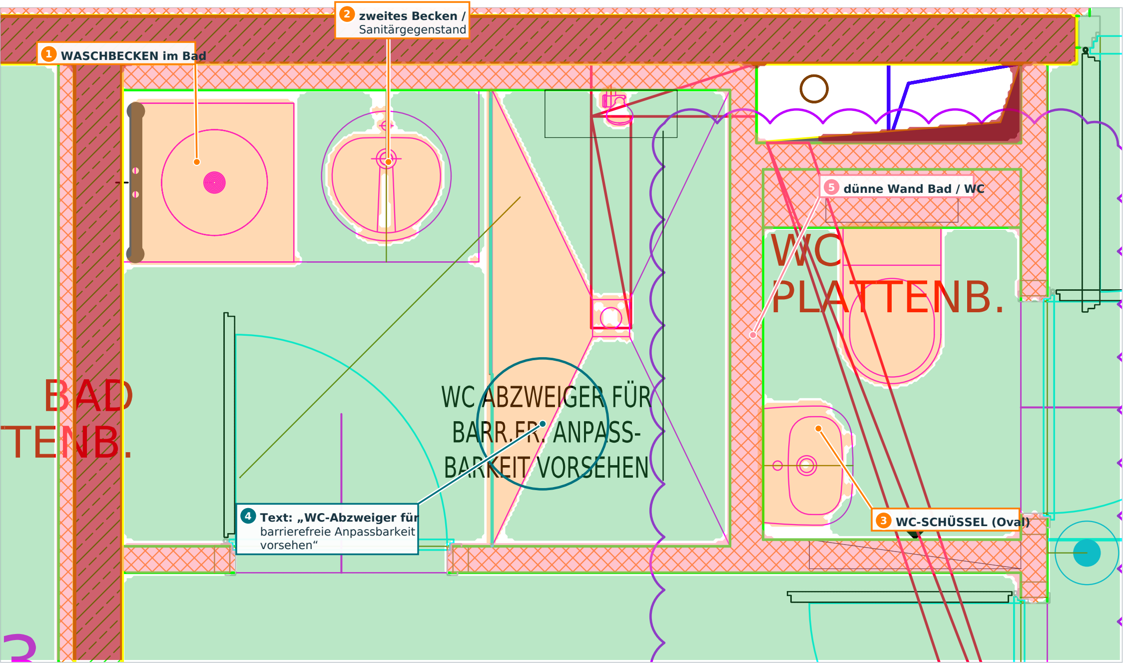
Hier bist du im Grundriss:
