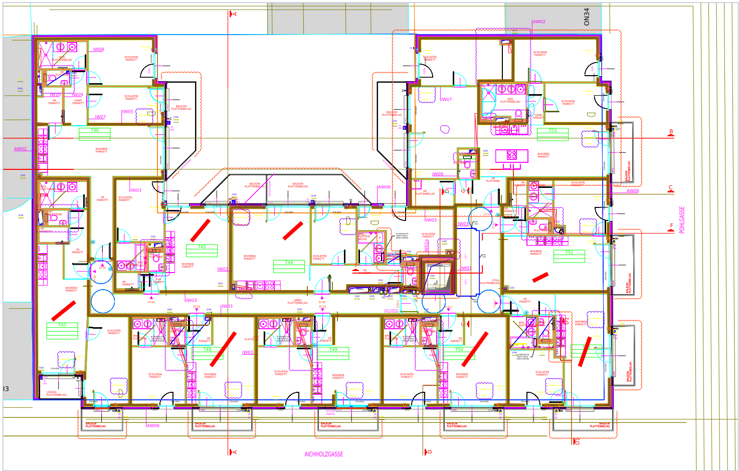
4. Obergeschoss (Wände rot)
