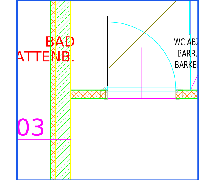
Lücke in der Wand + gerade Linie (Türblatt) + Viertelkreis (Öffnungsweg).
