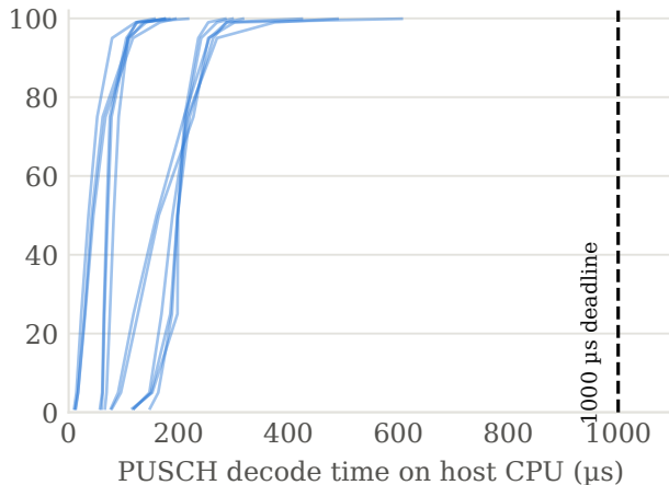
4G · 1 ms subframe
