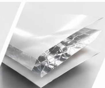
NY / ALU FOIL / PE
