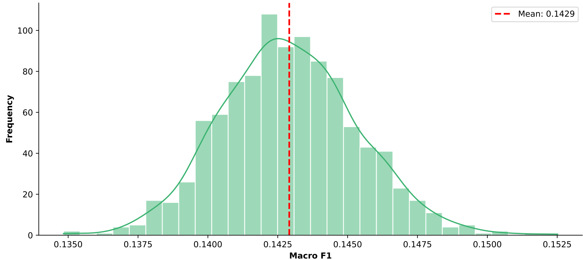
Random Classifier Macro F1 Distribution
