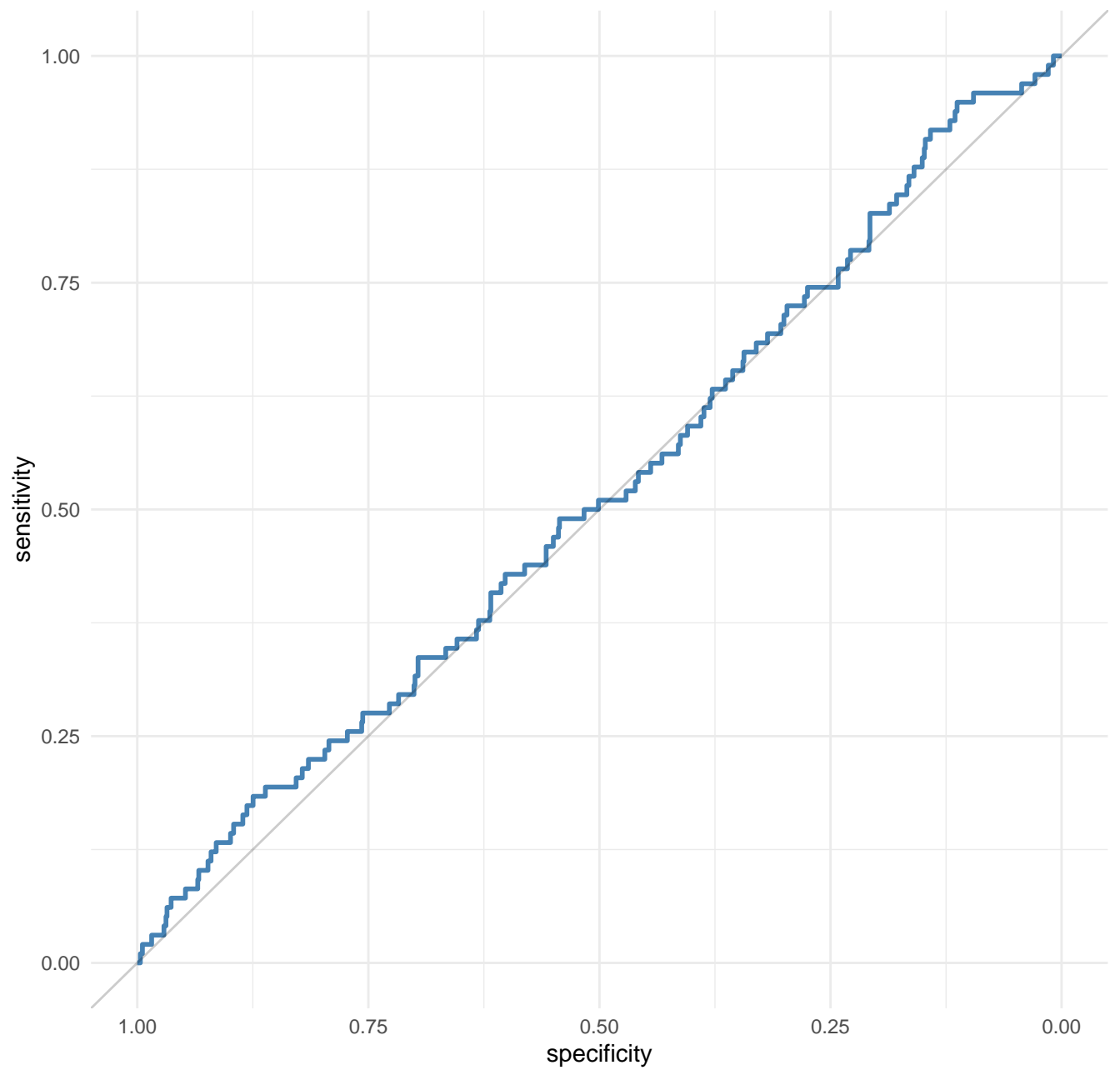
ROC curve (AUC = 0.5163)
