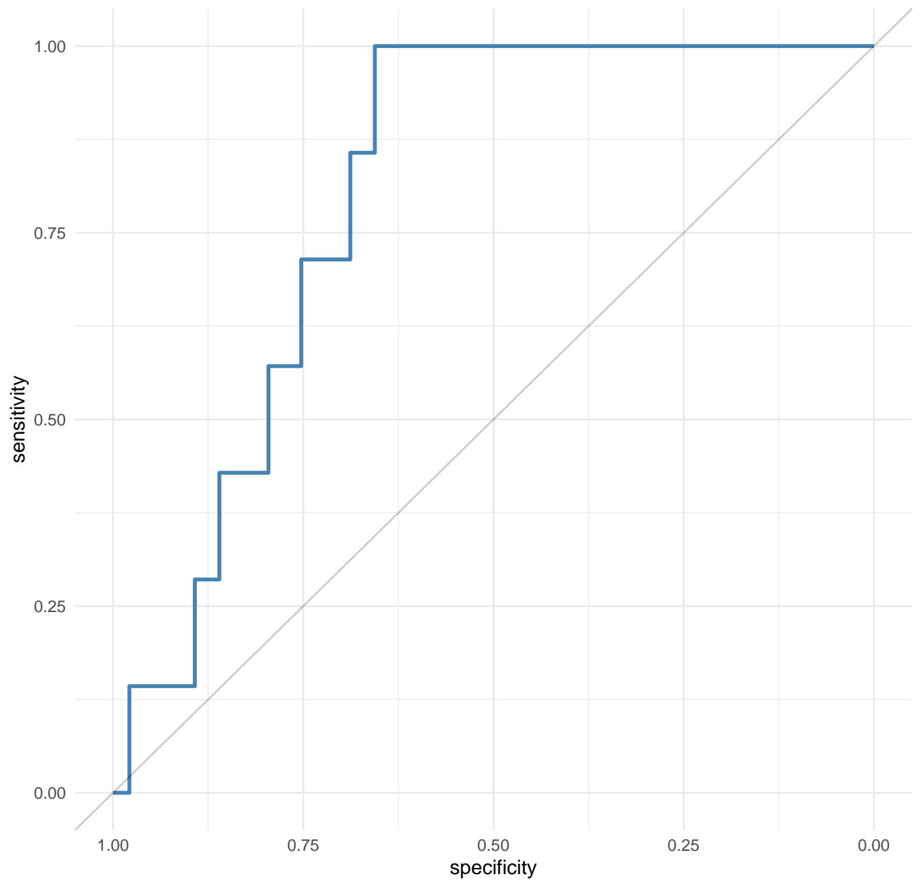
ROC curve (AUC = 0.8034)
