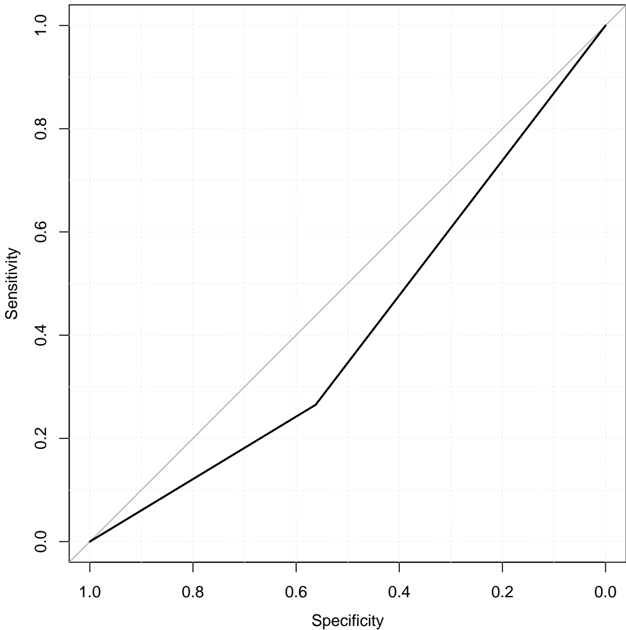
ROC curve (AUC = 0.4136)
