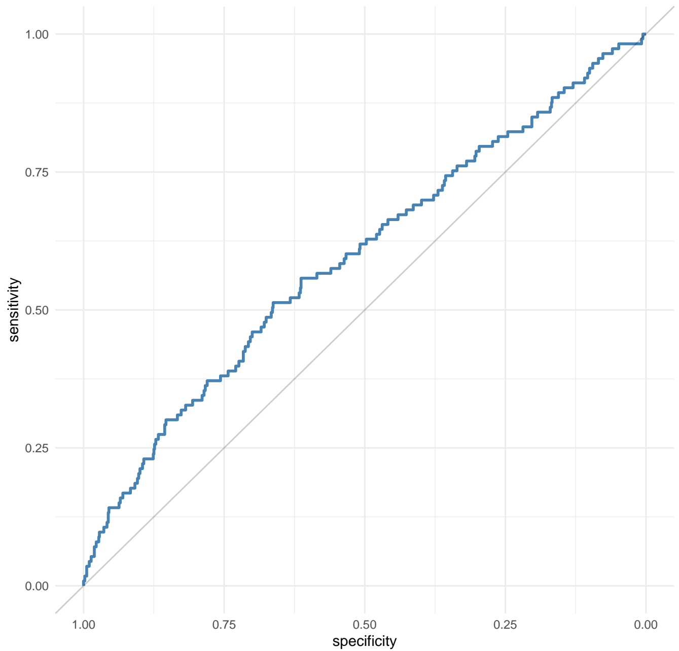
ROC curve (AUC = 0.5949)
