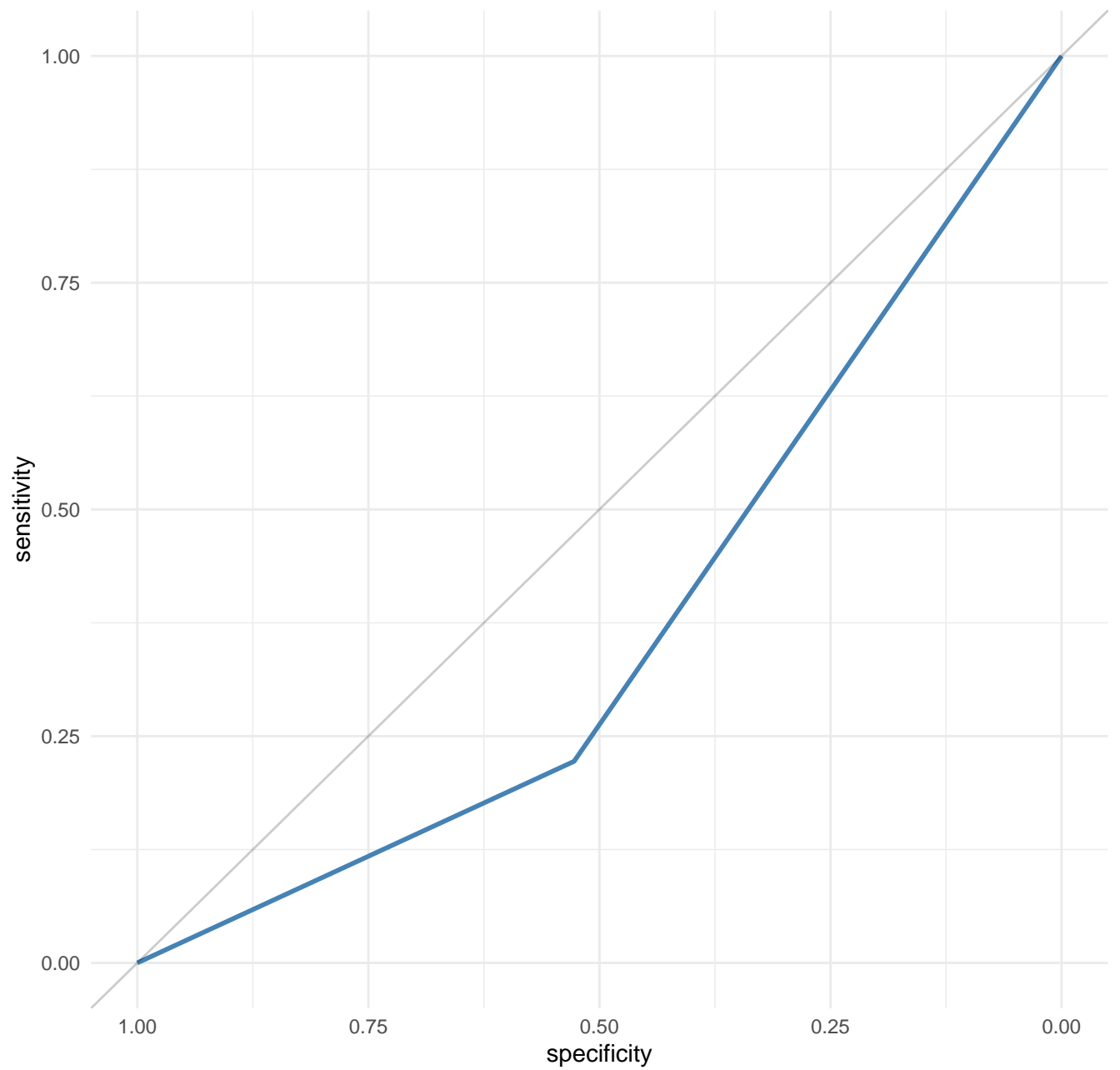
ROC curve (AUC = 0.3748)
