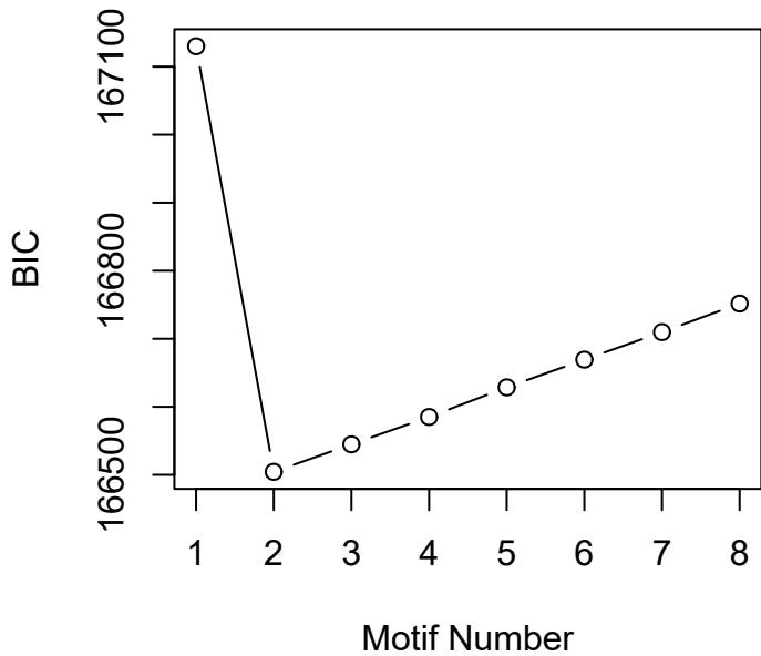
BIC
