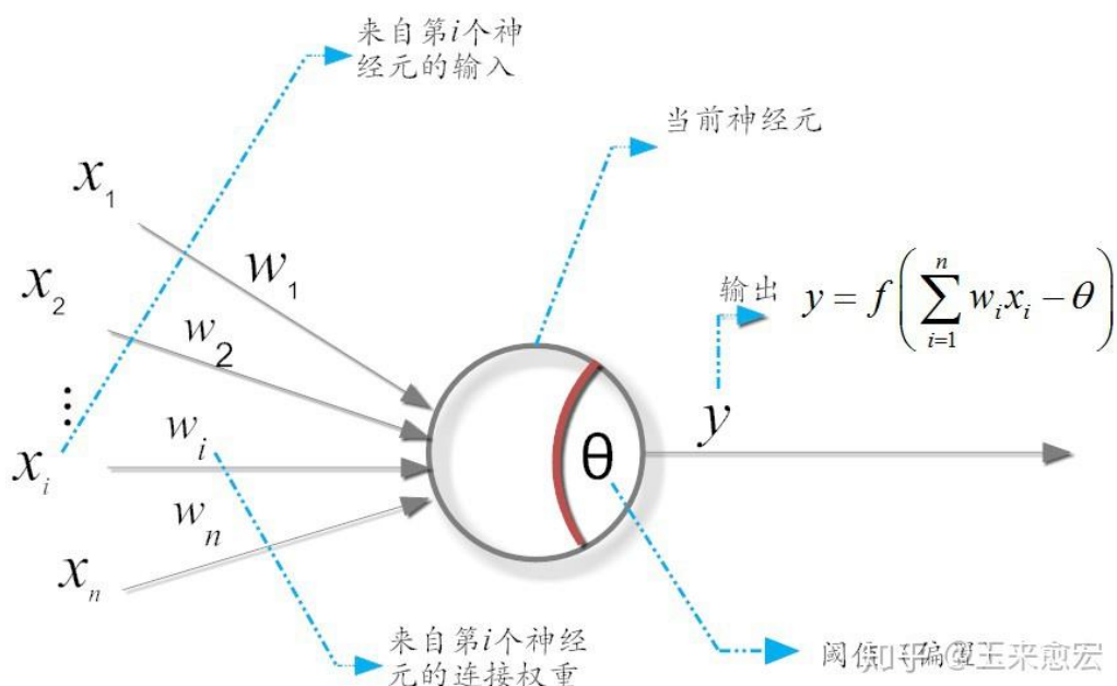
图 8.5: M-P 神经元模型：加权求和与阈值判定的二值输出。
