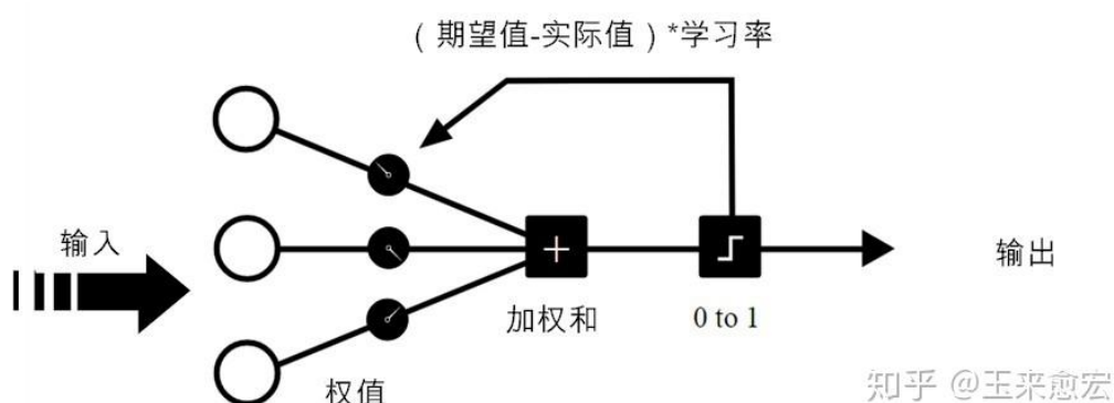
图 8.7: 罗森布拉特提出的感知机模型：引入基于误差反馈的参数学习机制。
