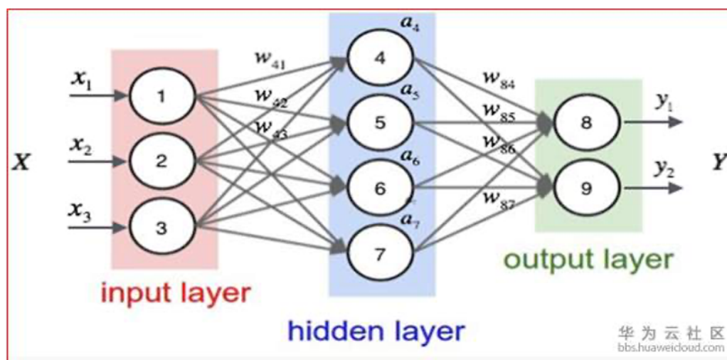
图 8.10: 多层感知机网络：通过隐含层实现非线性特征的分层抽象。
