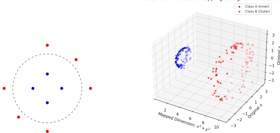
(a) 原始空间线性不可分的数据集
