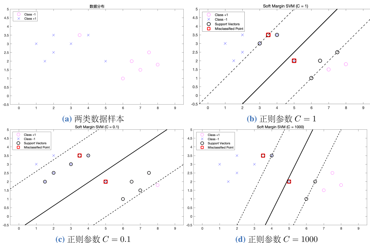
图 7.9: 软间隔 SVM 分类示例二
