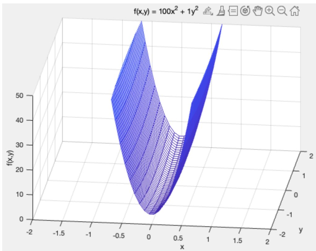
图 5.1: 参数为 a = 100, \varepsilon = 1 的二次峡谷曲面 f(x, y) = 100x^2 + y^2 : 梯度方向主要指向陡峭的横切面, 而非平缓的纵向延伸方向。
