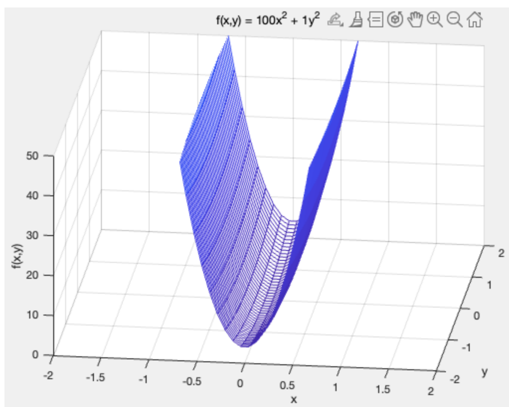
图 5.1: 参数为 a = 100 与 \epsilon = 1 的二次椭圆形抛物面
