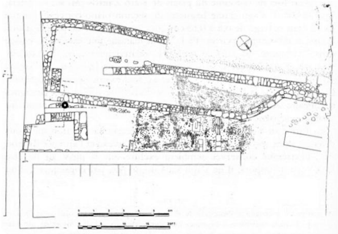
Fig. 1: Plan du péribole Sud-Ouest du palais (selon K. Tagonidou-Nakassi)
