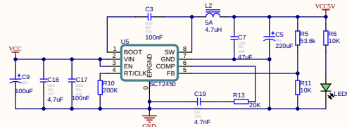
5V供电
