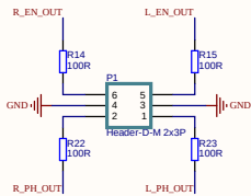
PH:对应PCB上DIR EN:对应PCB上PWM 电机信号接口
