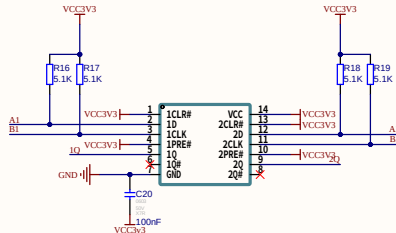
D触发器
