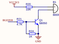
蜂鸣器
