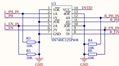
缓冲电路
