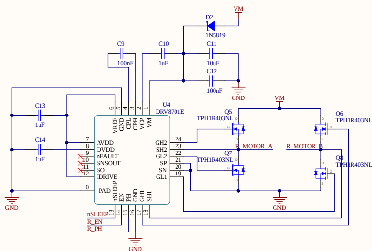
右电机驱动
