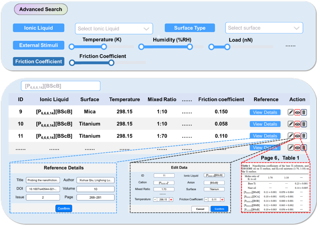
图 11: CILF-DB 数据检索与管理界面（上：高级检索模式，支持多维参数组合筛选；下：标准检索结果表格，含溯源窗口展开）
