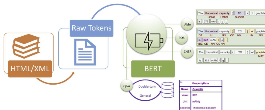
图 5: BatteryDataExtractor 系统架构与 NLP 流水线概述 [7] (HTML/XML 原始文本经 BERT 模型依次完成缩写检测、词性标注、化学命名实体识别和双轮问答提取, 最终输出结构化材料-性能数据库; 该系统明确指出”无法提取表格和图表中的信息”, 正是本研究引入 VLM 图表解析的直接动机)
