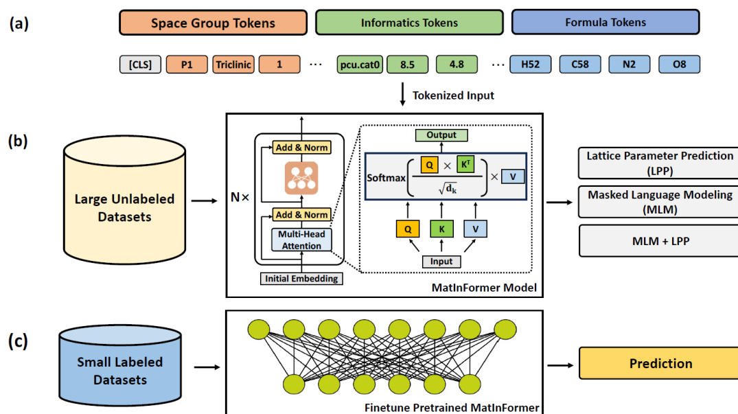
图 7: Materials Informatics Transformer (MatInFormer) 框架示意图 [7] ((a) 三类输入 Token: 空间群 Token 捕获晶体学对称性、信息 Token 编码 MOF 拓扑/孔隙率、化学式 Token 描述组成; (b) MLM+LPP 双策略预训练; (c) 下游材料属性预测微调; 该框架证明将材料知识编码为文本序列后 LLM 语义推理能力可迁移至材料性质预测, 为 CILF-DB 的 LLM 驱动数据提取提供方法论参照 [7, 7] )
