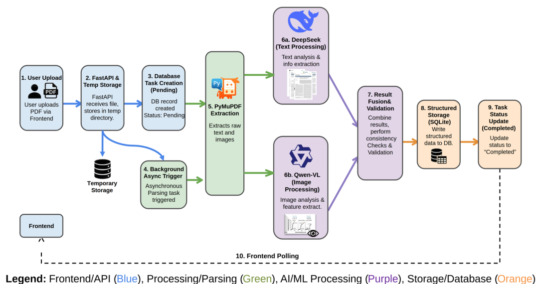
图 8: CILF-DB 平台完整数据处理流程图（蓝色：前端/API 层；绿色：解析处理层；紫色：AI/ML 提取层；橙色：存储层）
