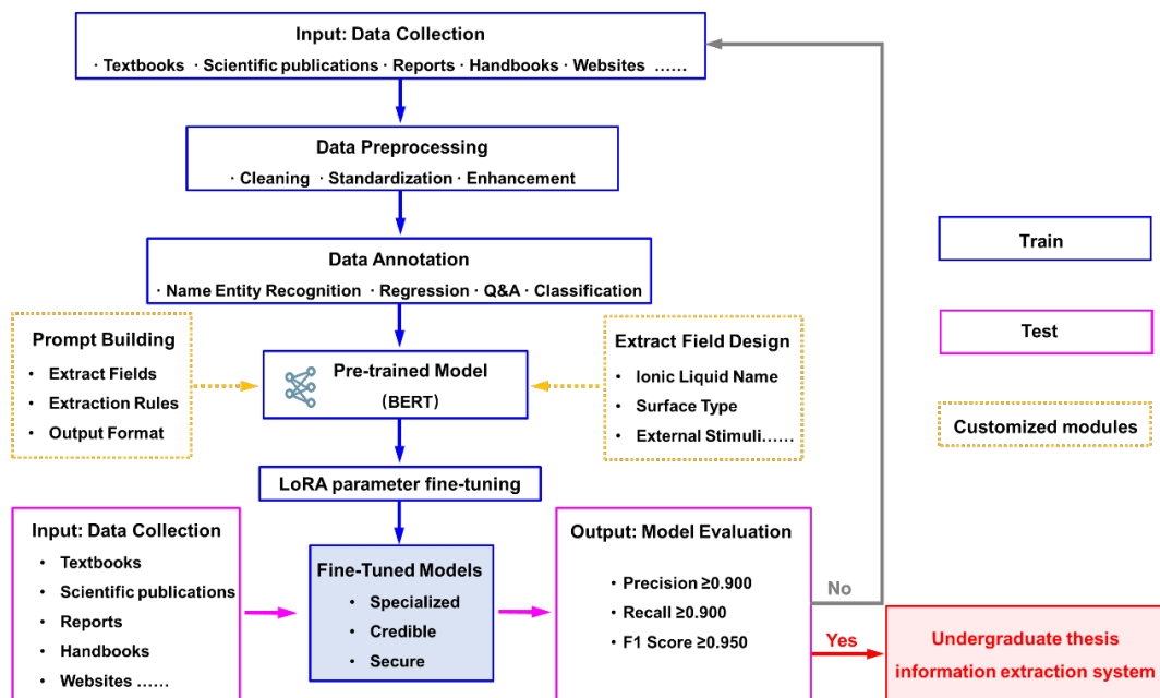
图 9: CILF-DB 平台 AI 模型训练与信息提取工作流（黄色虚线框为可定制模块；蓝色流程为训练路径，粉色流程为测试与部署路径）
