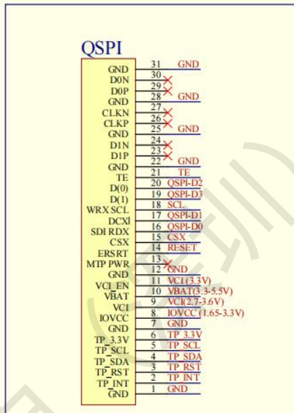
QSPI接口参考接线图
