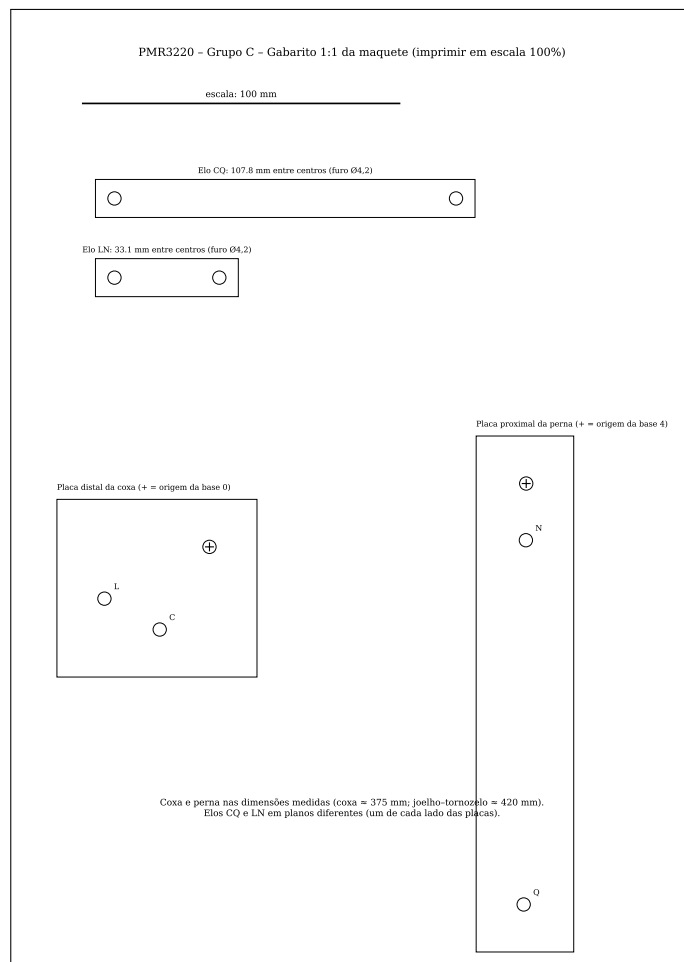
Figura 9: Gabarito da maquete (imprimir em escala 100%).
