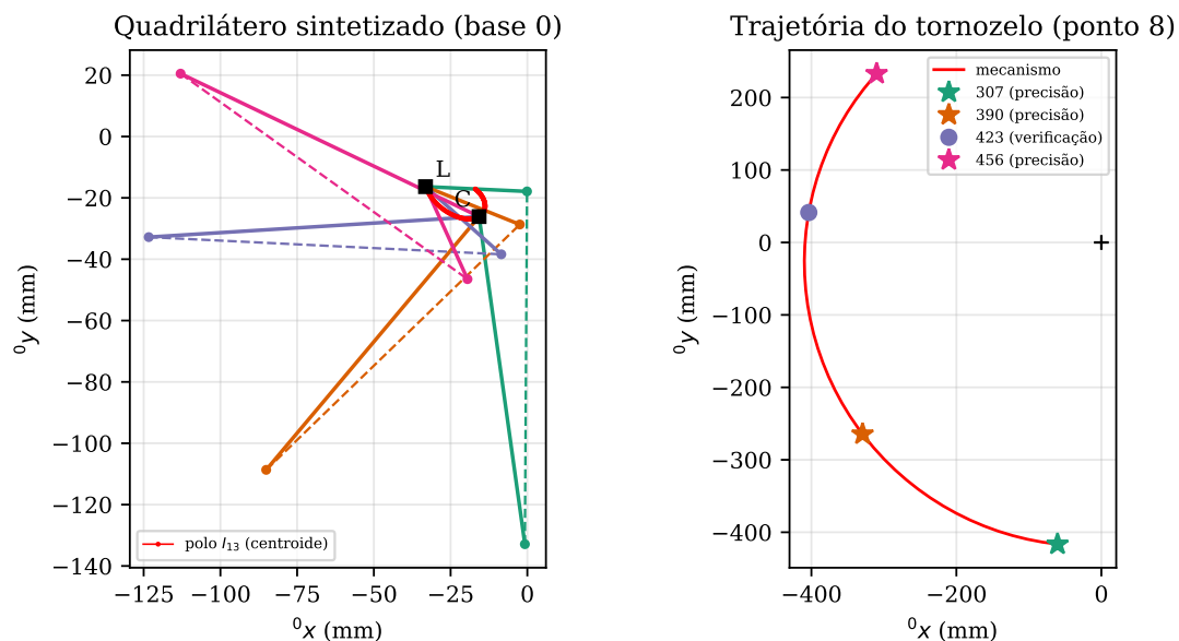
Figura 7: Esquerda: quadrilátero sintetizado nas quatro posições medidas (tracejado: acoplador QN ) e centroide. Direita: trajetória do tornozelo gerada pelo mecanismo e posições medidas.
