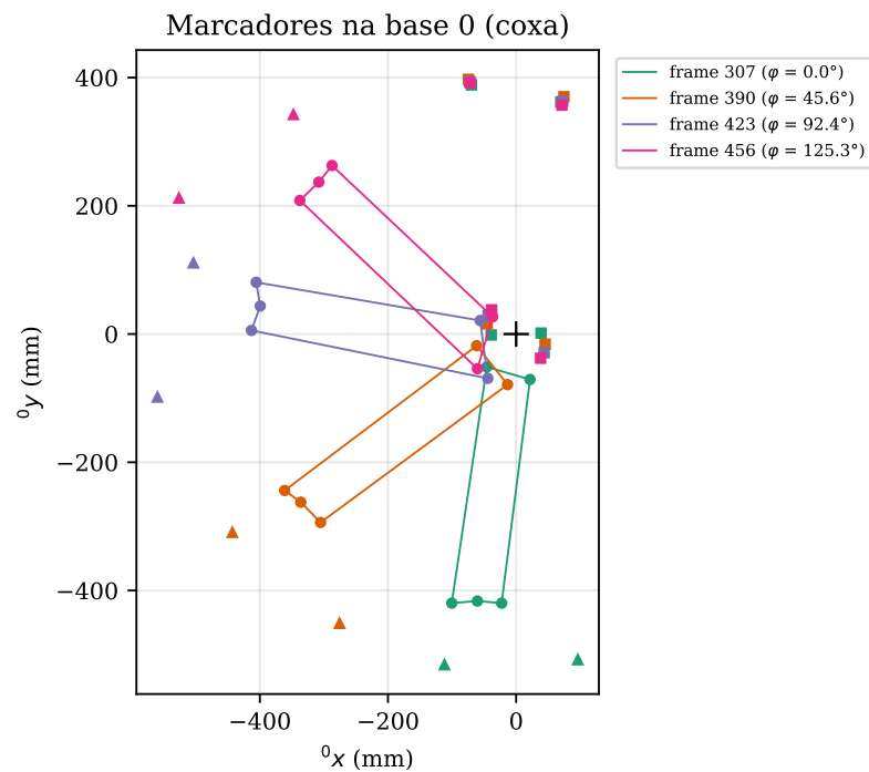
Figura 6: Marcadores dos quadros selecionados escritos na base da coxa ( \square : coxa, \circ : perna, \triangle : pé). A perna gira em torno da região do joelho enquanto a origem O_4 se desloca.
