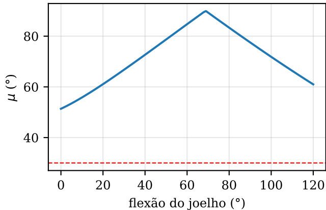
Ângulo de transmissão
