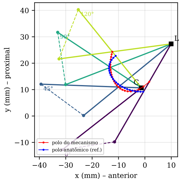
Quadrilátero sintetizado (referencial da coxa)
