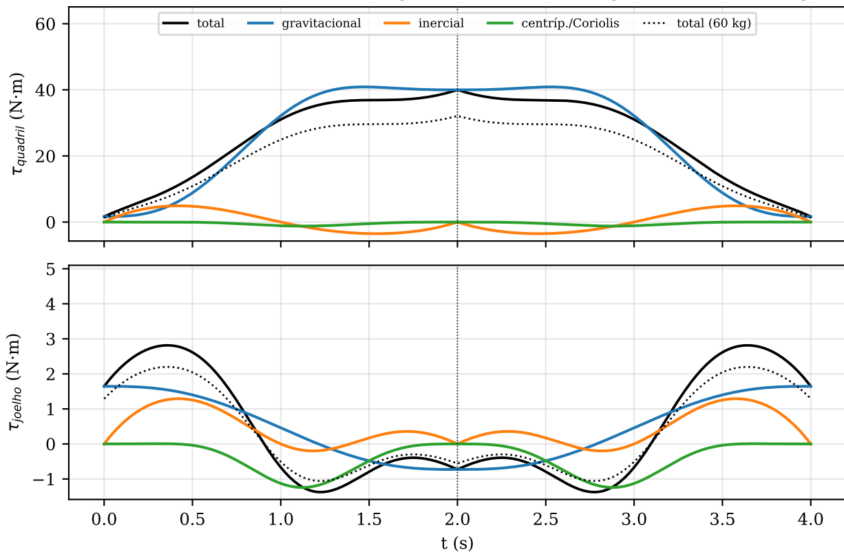
Torques dos atuadores - configuração final II (80 kg; pontilhado: 60 kg)
