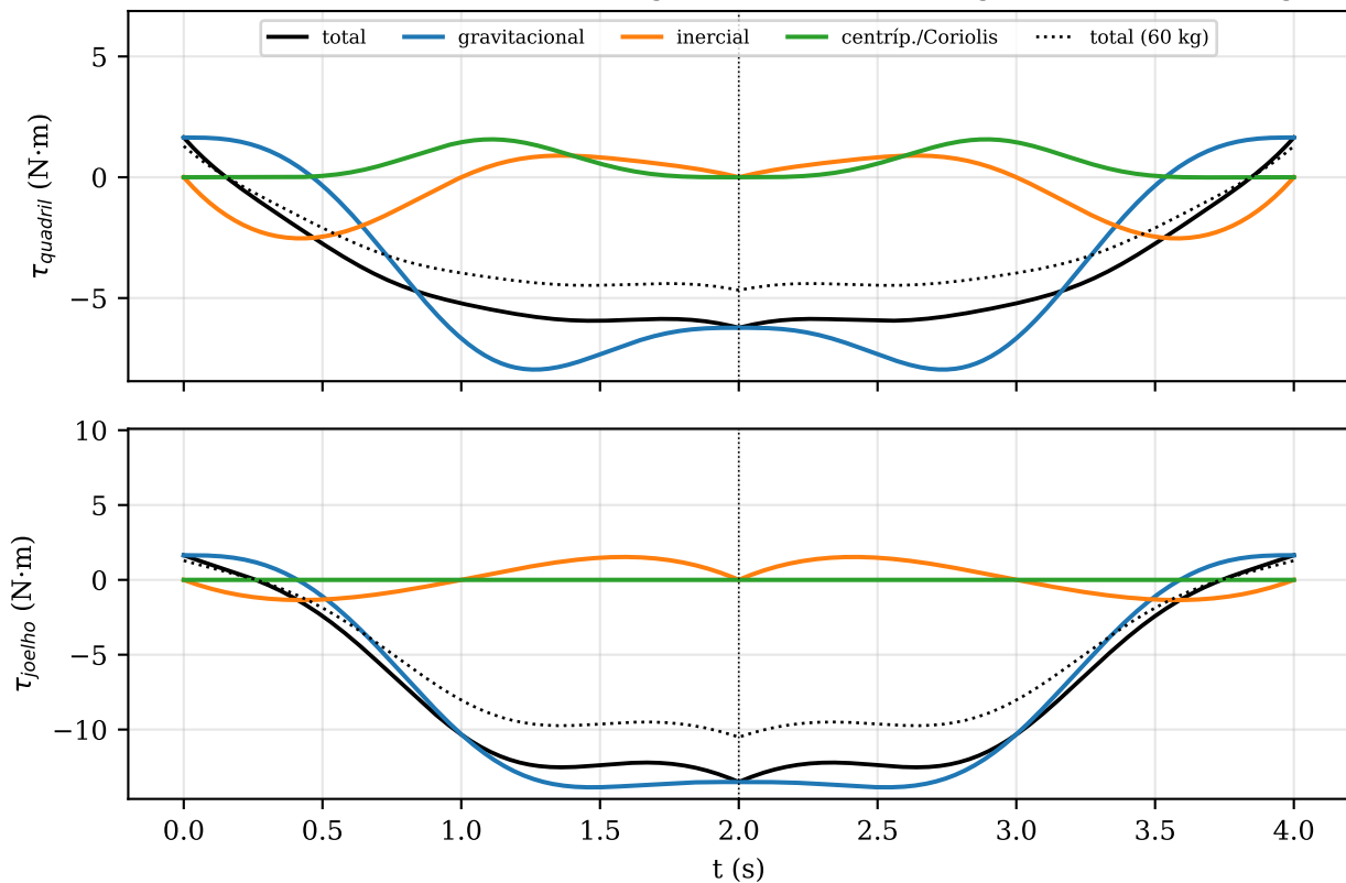
Torques dos atuadores - configuração final I (80 kg; pontilhado: 60 kg)
