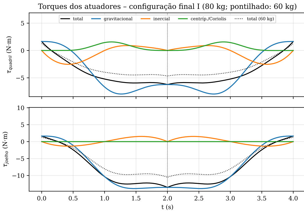
Figura 13: Torques no quadril e no joelho – configuração final I.
