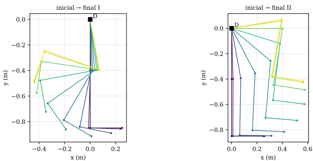
Figura 12: Instantâneos do movimento de ida (intervalos de T/8 ).
