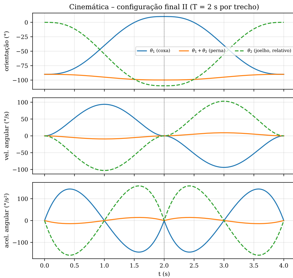
Figura 11: Orientação, velocidade e aceleração angulares – configuração final II.
