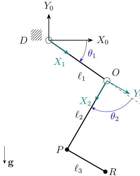
Figura 9: Cadeia aberta RR da órtese: bases 0 (fixa), 1 (coxa) e 2 (perna + pé). \theta_1 é medido de X_0 para X_1 e \theta_2 , de X_1 para X_2 (na figura, ambos negativos, isto é, no sentido horário).
