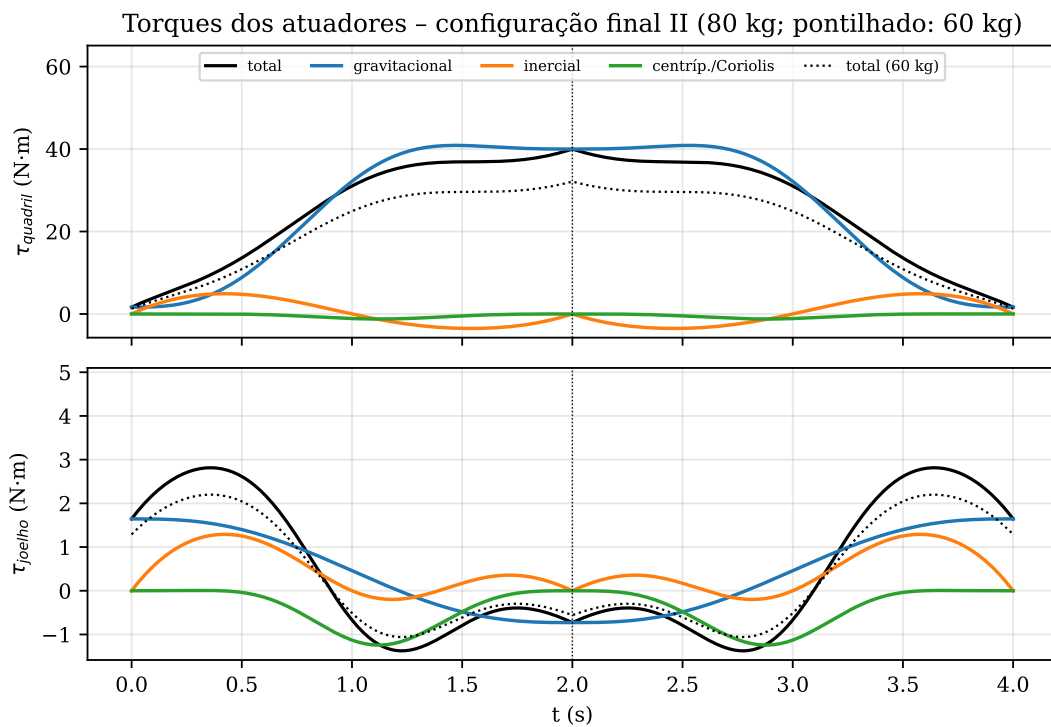
Figura 14: Torques no quadril e no joelho – configuração final II.
