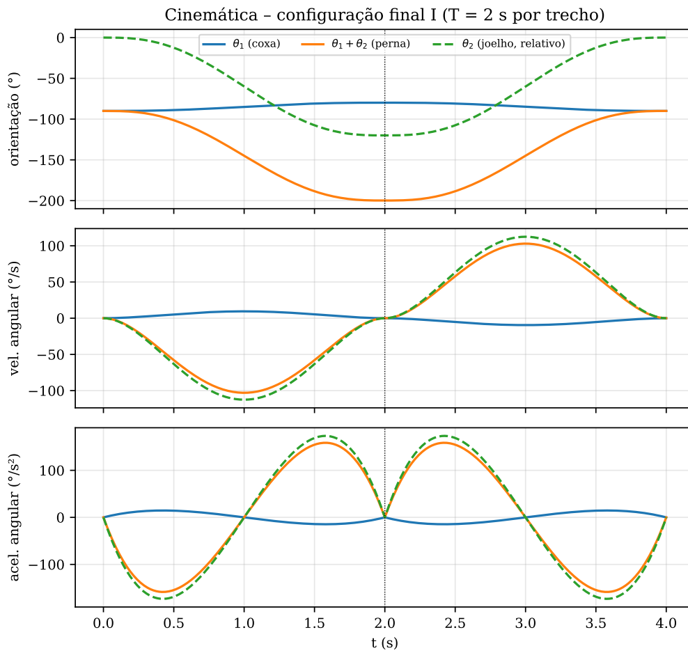
Figura 10: Orientação, velocidade e aceleração angulares – configuração final I.
