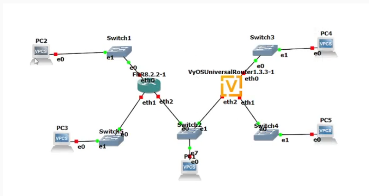
Рис. 2: Размещение устройств в соответствии с топологией.
