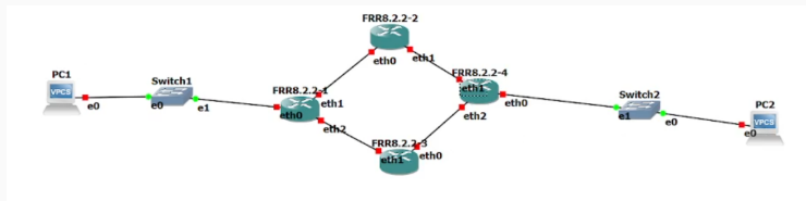
Рис. 2: Размещение устройств в соответствии с топологией.
