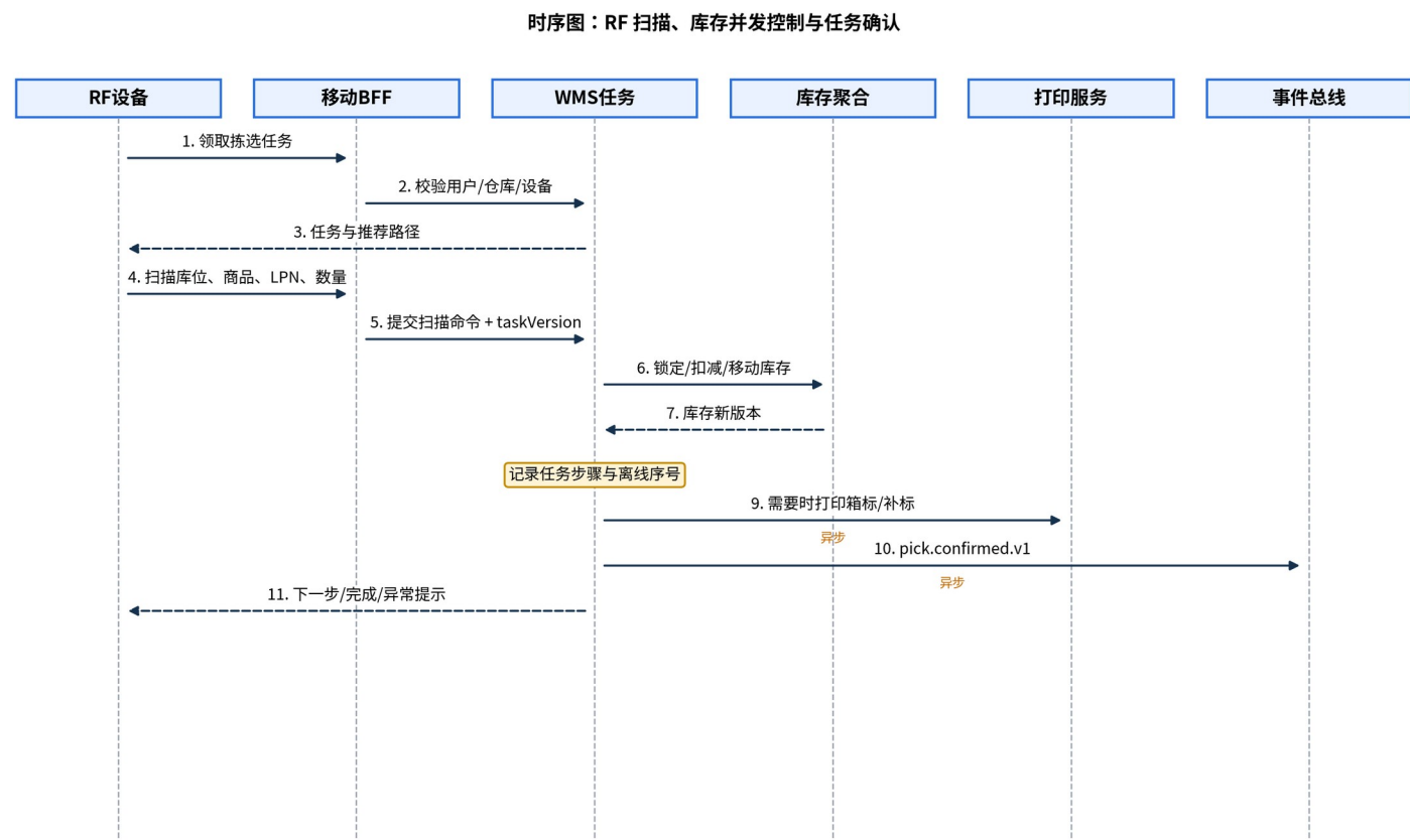
图 8-2 RF 扫描与库存并发
