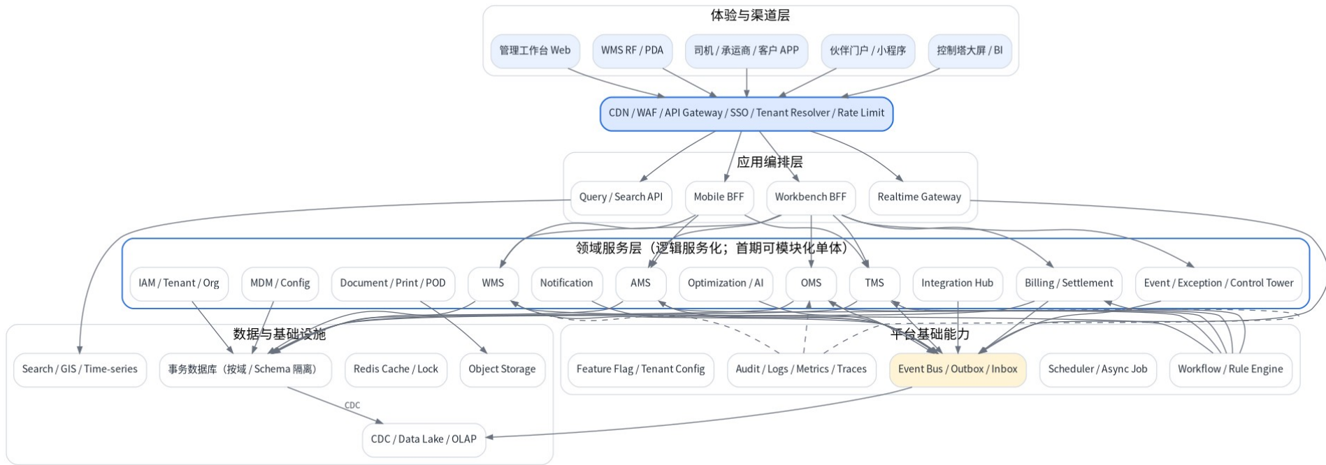
图 3-1 逻辑架构：渠道、编排、领域、平台基础能力和数据基础设施
