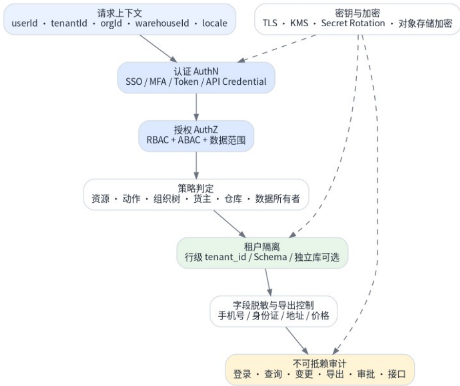
图 3-4 租户与安全：认证、RBAC+ABAC、数据隔离、脱敏、审计和密钥治理
