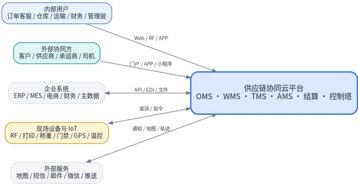
图 2-1 系统上下文：内部用户、合作伙伴、企业系统和设备围绕统一供应链平台协同
