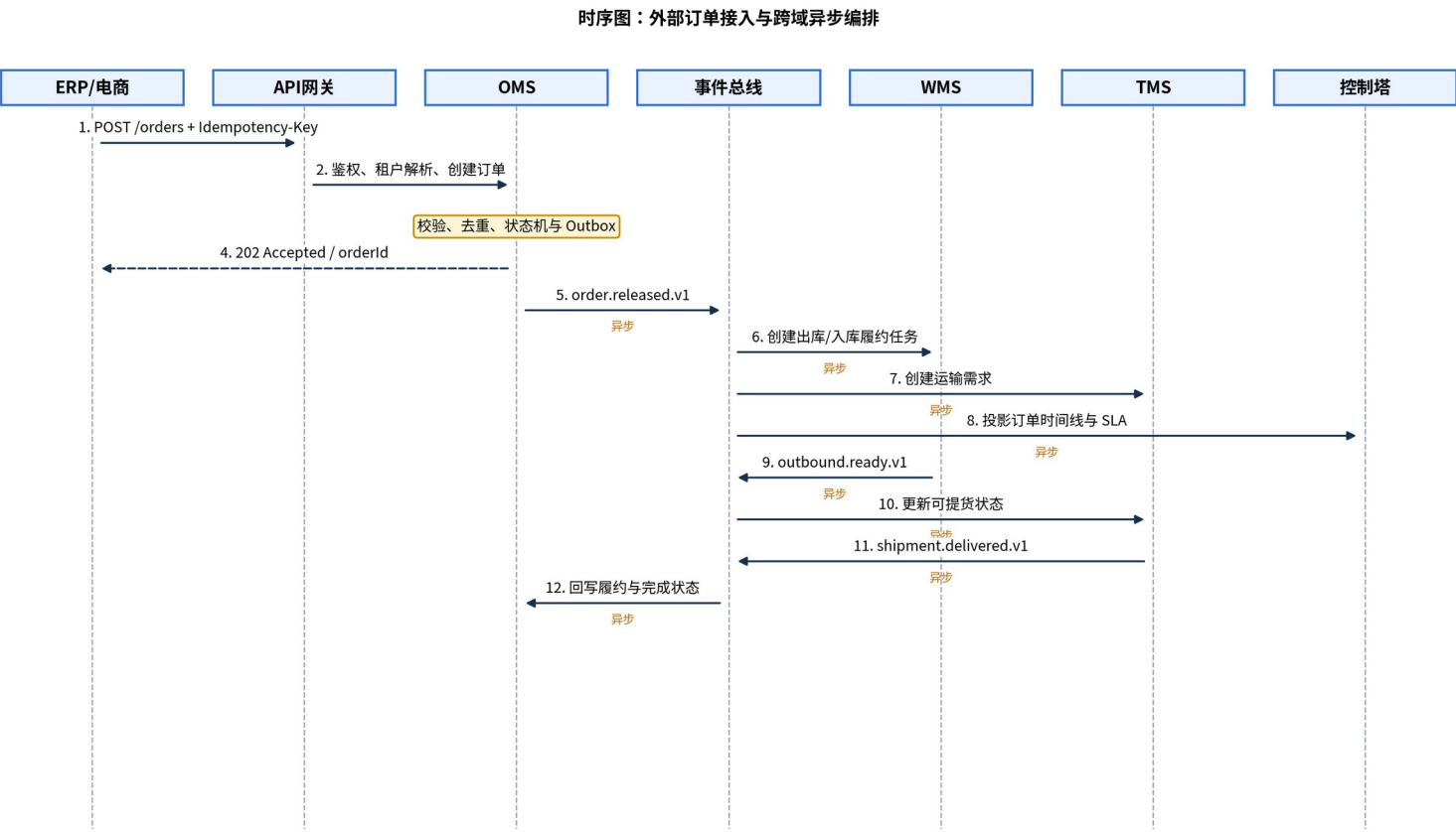
图 8-1 外部订单接入与跨域编排
