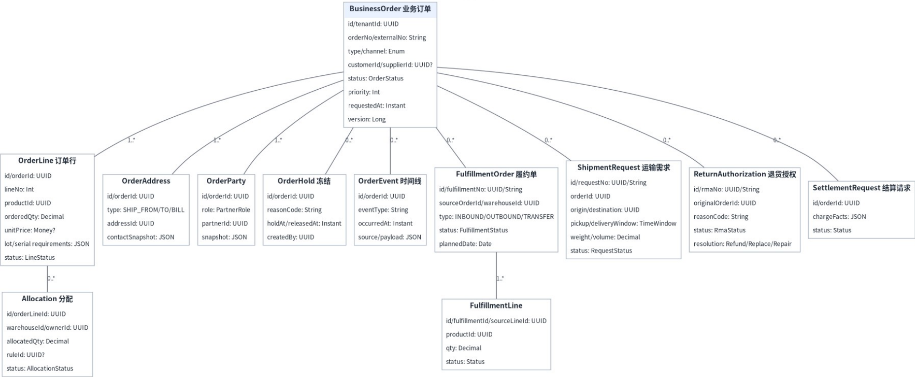
图 10-3 OMS 订单与履约类图
