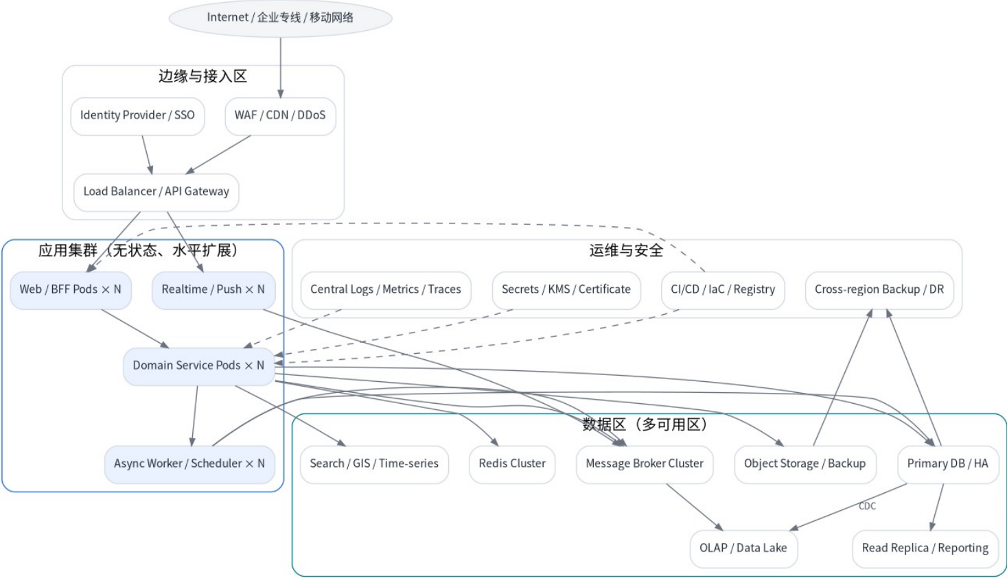
图 3-2 参考部署：边缘接入、无状态应用集群、多可用区数据层与运维安全
