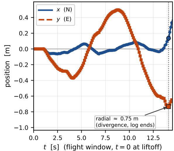
図 2 実機飛行（2026-06-22）における水平位置の時系列（横軸は離陸を原点とする時刻 t [s], 縦軸は位置 [m]）。飛行窓 14.5 秒のうちに動径方向の変位が 0.07 m から 0.75 m へ増大し、記録が終了した。
