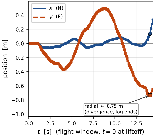
図2 実機飛行 (2026-06-22) における水平位置の時系列 (横軸は離陸を原点とする時刻 t [s], 縦軸は位置 [m]). 飛行窓 14.5 秒のうちに動径方向の変位が 0.07 m から 0.75 m へ増大し, 記録が終了した.
