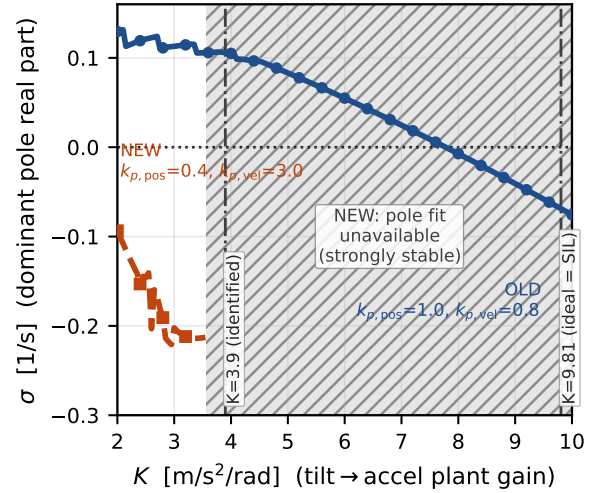
図3 線形カスケードモデルによる, 傾き→速度ゲイン K [\text{m/s}^2/\text{rad}] に対する支配極実部 \sigma [1/\text{s}] の掃引 (むだ時間 L = 150 \text{ ms} ). \sigma > 0 は不安定を示す. 旧ゲイン ( K_{p,\text{pos}} = 1.0 , K_{p,\text{vel}} = 0.8 ) は K/g \approx 0.64\text{--}0.80 を境に安定/不安定が入れ替わるのに対し, 新ゲイン ( K_{p,\text{pos}} = 0.4 , K_{p,\text{vel}} = 3.0 ) は掃引範囲全体で安定である.
