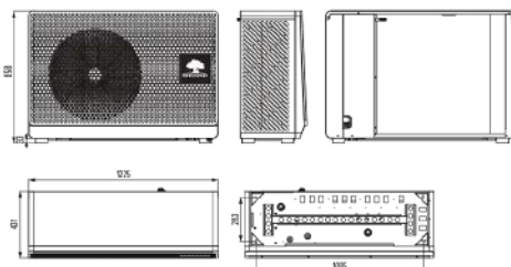
Зовнішній блок Вага 92кг
