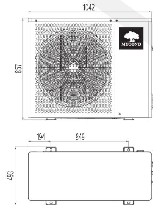
Тип MHS-U14/16BH (400В)
