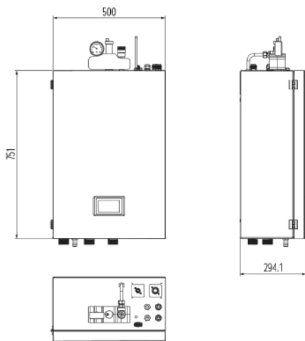
Внутрішній блок Вага 43кг
