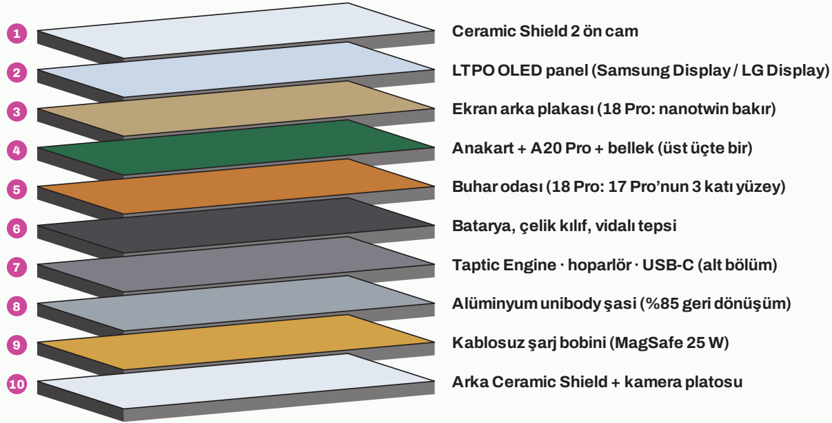
ŞEKİL 1 Özgün şematik çizim; ölçekli değildir. Katman sırası: iFixit iPhone 17 Pro teardown, 23 Eylül 2025. Rakamlar: Apple Newsroom 9 Eylül 2026; Apple AB Ürün Bilgi Formu A3714/A3717.
