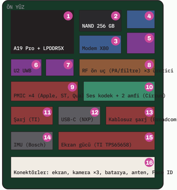
ŞEKİL 2 Özgün şematik; yonga konumları temsili, kodlar iFixit "iPhone 17 Pro Chip ID" (5 Kasım 2025) ve TechInsights 17 Pro Max teardown notundan.
