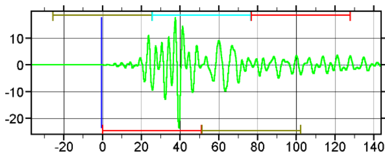
Obr. 1.2: Signál akustické emise pro vzdálenost senzoru od zdroje 6 cm [8]
