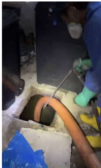
Proceso de limpieza y mantenimiento de tuberías y pozo séptico.
