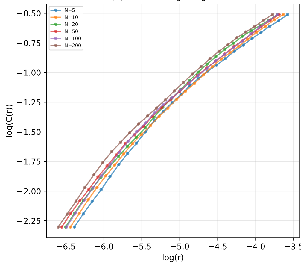
(d) G-P Scaling Diagnostic
