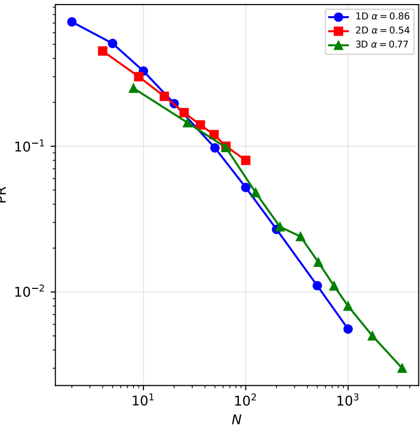
(d) All Dimensions
