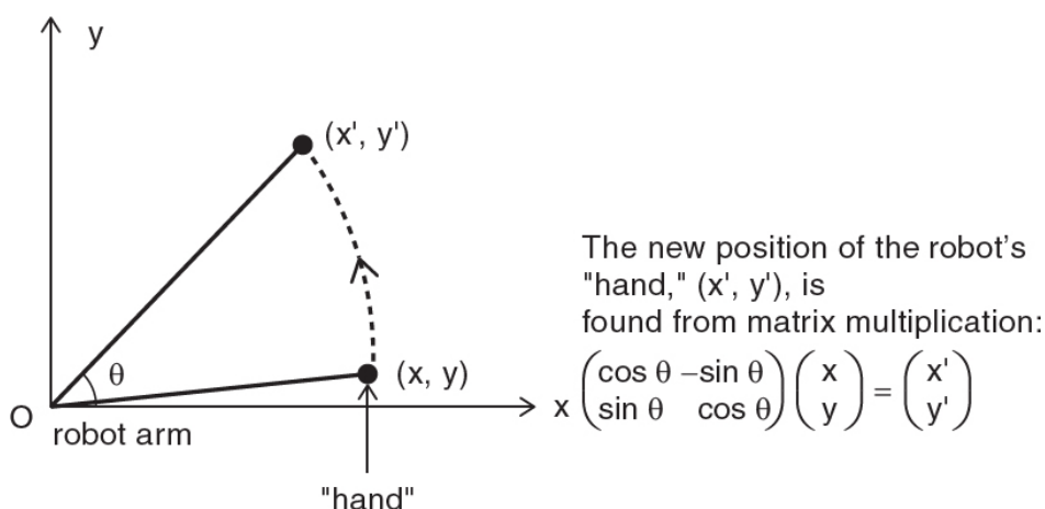
图 4.3: 绕 x - y 平面的原点、用旋转矩阵把一条机械臂逆时针转过角 \theta 。当你把这个矩阵方程的左端乘开，所得的那组方程——它说明如何用 x 和 y 写出 x' 与 y' ——就代表一个线性变换。不过这里的细节并不那么重要：关键是变换方程这个想法。
