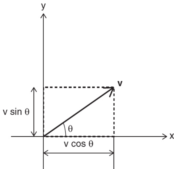
图 8.1 求抛射体的轨迹。球一旦被抛出，初速度为 v ，作用在它上面的唯一的力就是向下的重力。所以，在水平方向上没有力的分量。把这些分量分开来处理，先求运动的水平分量的值：在牛顿第二定律中消去质量项，并用牛顿的点记号表示时间导数，我们有： \ddot{x} = 0 \Rightarrow \dot{x} = C = v \cos \theta \Rightarrow x = vt \cos \theta 。（ C 是初速度的水平分量的大小；从原点抛出时，第二个积分常数为零。）现在求运动的竖直分量： \ddot{y} = -g \Rightarrow \dot{y} = -gt + C_1 = -gt + v \sin \theta \Rightarrow y = -\frac{gt^2}{2} + vt \sin \theta + C_2 （但从原点抛出时 C_2 = 0 ）。然后你就可以用 x 表示 t 并代入 y 的方程，从而得到那条抛物线轨迹。
