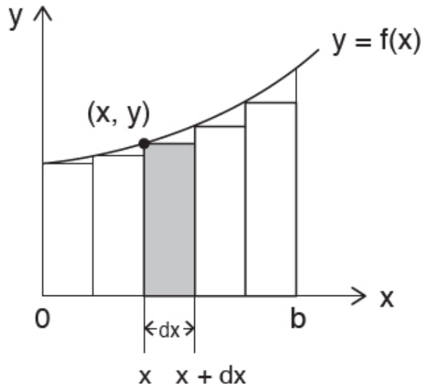
图 2.1 曲线下的面积。带阴影的矩形对应于图上一般的点 (x, y) ，它的面积（长乘宽）是 ydx 。当你对方程 y = f(x) 在 x = 0 与 x = b 之间“积分”时，你实际上是在求 dx 为无穷小时所有这些矩形的和。这个积分写作 \int_0^b ydx ，更具体地说，对于这个函数，是 \int_0^b f(x) dx ，它等于 x 轴与曲线 f(x) 之间、 x 取值在 0 与 b 之间的那块面积。
