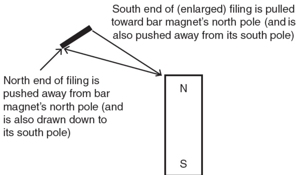
图 6.3B 使每一片铁屑（每一片都像一根小小的条形磁铁）排列起来的那些力。法拉第也对电做了同样的事情：在一个中心电荷周围的空间中各处放上一个小小的电“检验”电荷，并留意力在每个位置上如何作用。以这种方式，他构建出了电场与磁场的图景。（图内文字为英文，意为：铁屑的北极端被条形磁铁的北极推开，同时又被它的南极吸引；铁屑（放大后）的南极端被条形磁铁的北极吸引，同时又被它的南极推开。）
