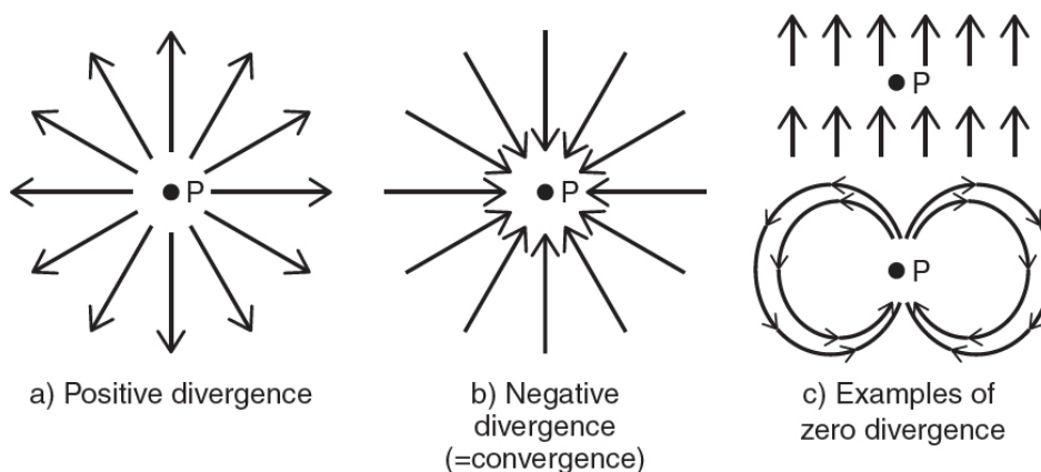
图 7.1 散度。举个例子, 库仑定律告诉我们: 如果在 P 处有一个带正电的粒子, 而你把单位正试探电荷放在 P 周围场中的不同位置上, 那么电力的方向就如图 (a) 中的箭头所示。随着你远离 P , 力按平方反比定律衰减, 所以箭头会变小。如果试探电荷是负的, 它会被 P 处的正电荷吸引, 于是你就得到了情形 (b)。在《电磁通论》( Treatise on Electricity and Magnetism ) 第 1 卷 (第 77 节) 中, 麦克斯韦借助高斯关于库仑定律与通量相关的想法, 把这个定律写成 \frac{\partial X}{\partial x} + \frac{\partial Y}{\partial y} + \frac{\partial Z}{\partial z} = 4\pi\rho , 其中方程的左边是电力的散度 (他把它分量写作 X, Y, Z ), 而 \rho 是场的电荷密度。我在第 6 章的一条尾注中说明过麦克斯韦是如何利用通量的想法推导出这个方程的。(c) 中下面那幅图看上去像条形磁铁周围的力线, 如图 6.3a 所示——而我们后面会看到, 麦克斯韦的又一个方程说的是磁场的散度为零。(图内三个面板的标题为英文: a) Positive divergence = 正散度; b) Negative divergence (=convergence) = 负散度 (=收敛); c) Examples of zero divergence = 零散度的例子。)
