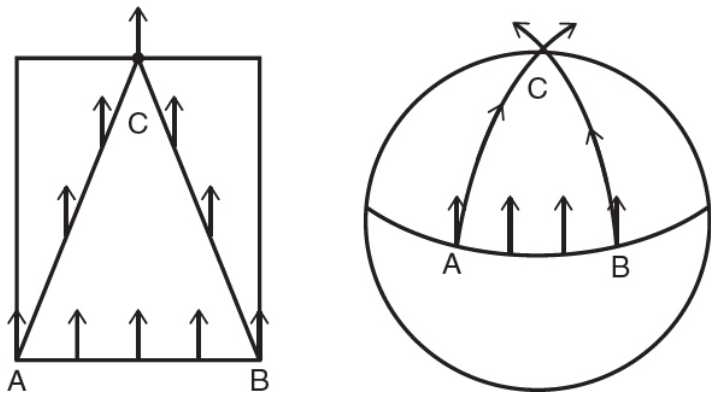
图 13.2: 把一个从点 A 出发时是竖直的向量作平行移动 (parallel transport)，在平坦空间中毫无问题——但在曲面上，这个概念必须被仔细定义。我在相关的知识框里对此多解释了一点。
