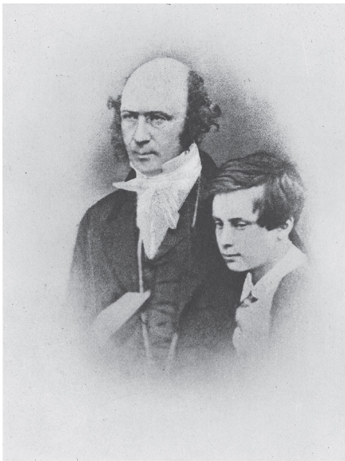
图 4.1: 威廉·罗恩·哈密顿爵士与他的一个儿子（约 1845 年）；经皇家爱尔兰学院许可使用 © RIA。在那个年代，拍照需要很长的曝光时间，这大概解释了为什么照片上的哈密顿从来不笑；不过大家都说，他极富幽默感。
