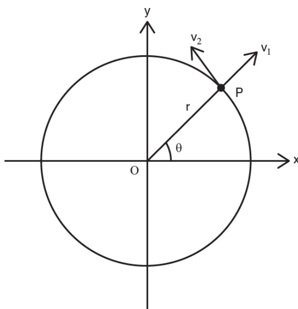
图 0.3: 半径为 r 的圆上一点 P 的极坐标；角度 \theta 按逆时针方向度量。速度分量分别沿 r 方向、以及 \theta 增大的方向度量，如图所示。
