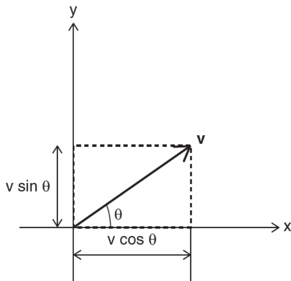
图 8.1: 求抛射体的轨迹。球一旦被抛出，初速度为 v ，作用在它上面的唯一的力就是向下的重力。所以，在水平方向上没有力的分量。把这些分量分开来处理，先求运动的水平分量的值：在牛顿第二定律中消去质量项，并用牛顿的点记号表示时间导数，我们有： \ddot{x} = 0 \Rightarrow \dot{x} = C = v \cos \theta \Rightarrow x = vt \cos \theta 。（ C 是初速度的水平分量的大小；从原点抛出时，第二个积分常数为零。）现在求运动的竖直分量： \ddot{y} = -g \Rightarrow \dot{y} = -gt + C_1 = -gt + v \sin \theta \Rightarrow y = -\frac{gt^2}{2} + vt \sin \theta + C_2 （但从原点抛出时 C_2 = 0 ）。然后你就可以用 x 表示 t 并代入 y 的方程，从而得到那条抛物线轨迹。
