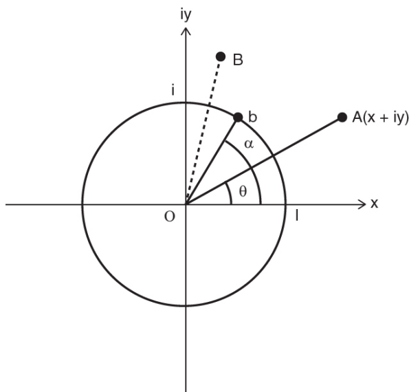
图 4.4: 旋转一个复数的“机械装置” (参看图 3.8)。把点 A 表示为复数 x + iy = r \cos \theta + ir \sin \theta = re^{i\theta} 。要把 OA 绕原点转过一个角 \alpha ，就用单位复数 b = ei\alpha 去乘它，得到新的点 B = (ei^\alpha)(x + iy) = (ei^\alpha)re^{i\theta} = re^{i(\theta+\alpha)} 。(如果你只想旋转原来的向量、而不想同时改变它的长度，那么这个“机械装置”就必须是一个单位向量，就像图 3.8 那样。)
