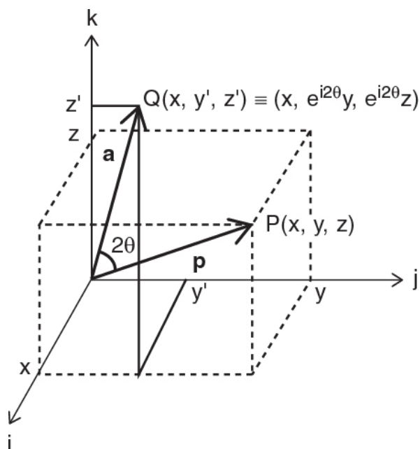
图 4.5: 用四元数做三维旋转。当 \mathbf{p} = ix + jy + kz 绕 i 轴转过角 2\theta 时，它的新位置向量是 \mathbf{a} = xi + ei^{2\theta}(yj + zk) 。我之所以为这个角选取 2\theta 而不是 \theta ，是因为它将与量子力学有一段有趣的关联，我们很快就会看到。
