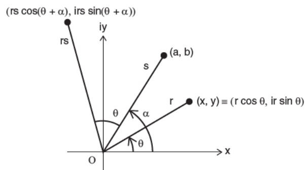
图 3.9: 如何通过旋转来计算乘法: 利用极坐标和欧拉公式写出 x + iy = r \cos \theta + ir \sin \theta = re^{i\theta} , 以及 a + ib = s \cos \alpha + is \sin \alpha = se^{i\alpha} ; 然后利用指数律, 你会看到乘积是 rse^{i(\theta+\alpha)} 。所以, 用 a + ib 去乘 x + iy , 是把原向量的模拉长了, 并把它旋转了 \alpha 弧度。而单纯地把一个复数加到另一个上, 则可以看作平面中的一次平移。
