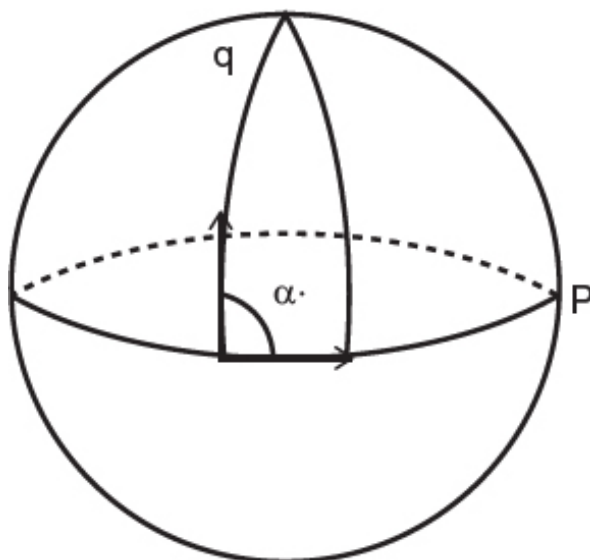
图 10.5: 一个由三条大圆坐标线围成的球面三角形。两条这样的线之间的夹角, 就是它们切向量之间的夹角, 如箭头所示。在球面上, 三个角都是直角。
