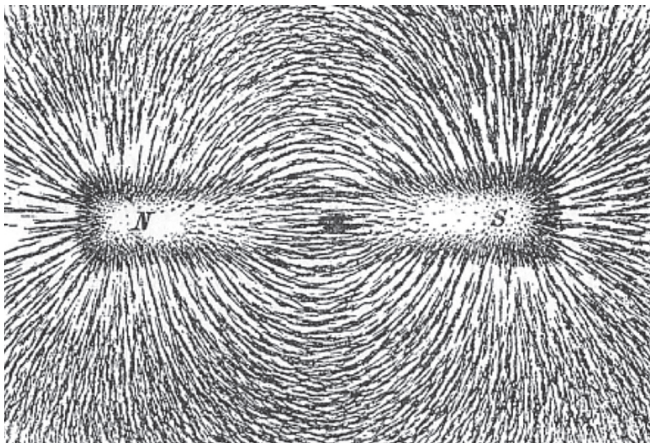
图 6.4: 铁屑在一块磁铁周围排列成行。Newton Henry Black 与 Harvey N. Davis, 《实用物理学》( Practical Physics ) (纽约: Macmillan, 1913 年)。维基共享资源, 公有领域。
