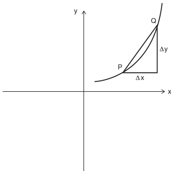
图 2.5: 直线 PQ 的斜率是 \frac{\Delta y}{\Delta x} ；它逼近 P 与 Q 之间那段图像的梯度。要说得更专业——也更现代——一些，我们需要极限：为了得到 P 处的精确梯度——并由此求出 P 处的导数——你把点 Q 越来越接近地移向 P，直到 \Delta x 与 \Delta y 都变成无穷小。于是图像在 P 处的导数，就是当 \Delta x \rightarrow 0 时 \frac{\Delta y}{\Delta x} 的极限。取了极限之后，莱布尼茨的记号 \frac{dy}{dx} 就取代了 \frac{\Delta y}{\Delta x} 。如果你拿到的是一幅距离 x 对时间 t （而不是如图所示的 y 对 x ）的图像，那么梯度——这时是 \frac{dx}{dt} ——就代表速率 v ——即单位时间内的距离。
