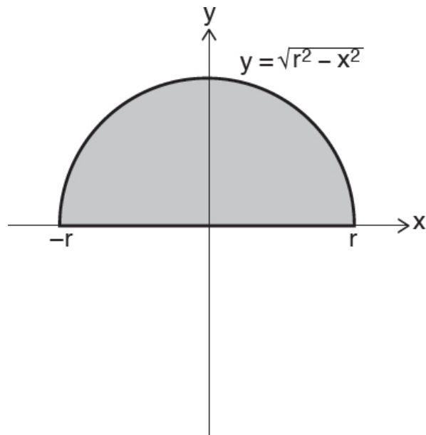
图 2.3: 用积分学求圆的面积。思路是求出半圆 y = \sqrt{r^2 - x^2} 下方的面积，再乘以 2。
