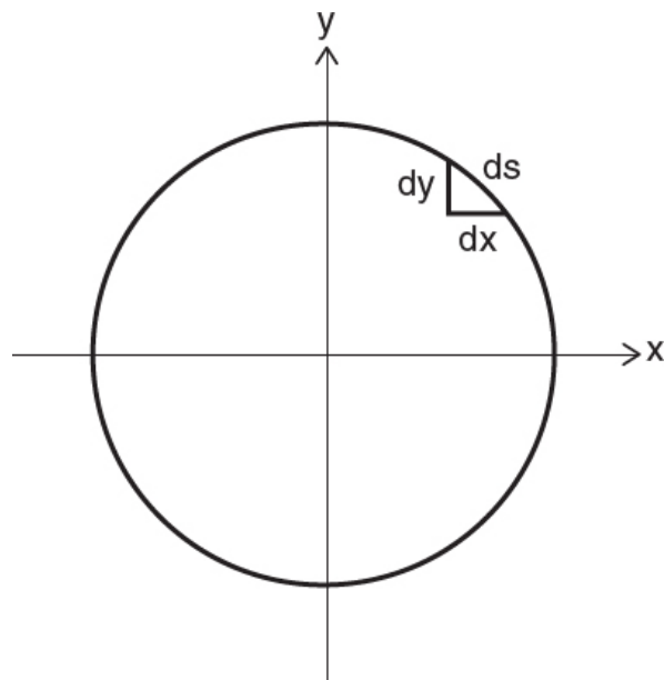
图 2.4: 用积分学求圆的周长。这里的思路是把所有那些小段 ds 加起来（积分！）。（我会在相关的知识框里给出部分计算，不过在这里，也像全书其他地方一样，如果细节不是你的菜，我希望你不要就此停下不读，而是直接跳过去，继续往下看故事。）
