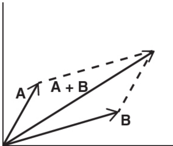
图 3.1: 把两个向量 A 与 B 相加。牛顿和使用平行四边形的其他早期先驱，在这里大概并没有想着要把向量或“线”相加，但我们今天正是这样理解的： A 与 B 是合成向量 A + B 的分量。平行四边形法则的一个关键特征是，在这样的向量和中，两个分量各自独立地起作用，意思是每一个的表现都仿佛另一个并不在场。换句话说，当你用平行四边形法则把两个分量相加时，你并不改变它们原本的大小或方向，只是把它们平移过去，构成平行四边形的两条对边。
