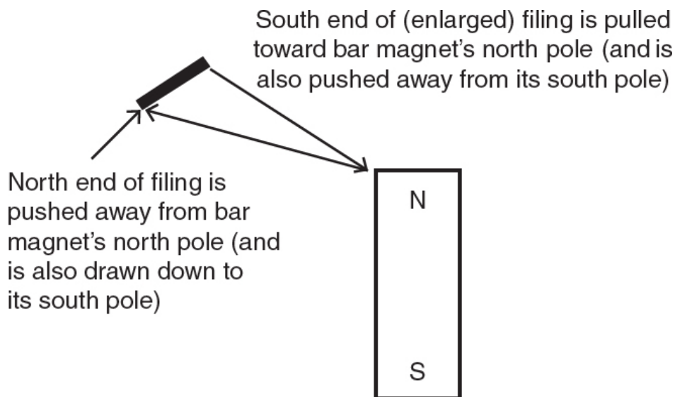
图 6.5: 使每一片铁屑（每一片都像一根小小的条形磁铁）排列起来的那些力。法拉第也对电做了同样的事情：在一个中心电荷周围的空间中各处放上一个小小的电“检验”电荷，并留意力在每个位置上如何作用。以这种方式，他由此构建出了电场与磁场的图景。
