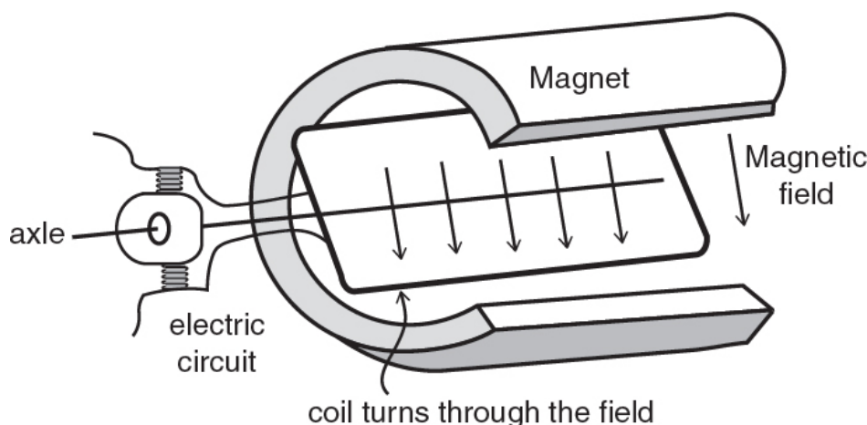
图 6.3: 电动机与发电机: 正如奥斯特发现的那样, 电流可以产生磁力; 而且人们早已知道两块磁铁会相互吸引或排斥 (异极相吸)。所以, 当一个载流线圈被置于一个外部磁“场”中——这里用磁极之间的箭头表示——它自身的磁场就会与外部磁场相互作用。这使线圈发生偏转并转动起来——而这种转动效应 (力矩) 在电动机中得到了利用。随着线圈转动, 它与外部磁场所成的角度在变化——这意味着穿过线圈的磁通量在变化 (参看图 6.1)。所以, 如果你先用机械方式转动这个环, 那么穿过环的变化着的磁通量就会感生出产生电流所需的电磁场——而这正是发电机的基础。
