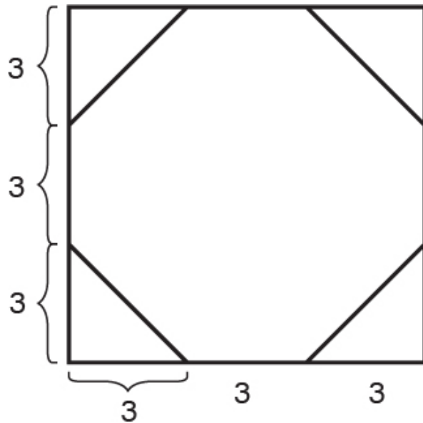
图 2.2: 古埃及对圆的面积与周长的估算。正方形边长为 9 个单位，所以它的面积是 81 平方单位。内接八边形的面积 = 正方形面积减去四个角上三角形的面积 = 81 - 4 \left( \frac{3 \times 3}{2} \right) = 63 平方单位。这看起来已经很接近 64 平方单位了，而 \sqrt{64} 比 \sqrt{63} 容易对付得多——于是阿赫摩斯把这个圆的面积记作等价于一个边长为 8 单位的正方形的面积。由于八边形被当作原正方形内切圆的近似，这个圆的半径就是 \frac{9}{2} 个单位。所以他们的面积公式(用现代术语说)是 A = Nr^2 ，其中 N 代表他们那个版本的 \pi : N = \frac{A}{r^2} = \frac{64}{(\frac{9}{2})^2} = 64 \times \frac{4}{81} = \frac{256}{81} ，约等于 3.16；现代值是 3.14 稍多一点。
