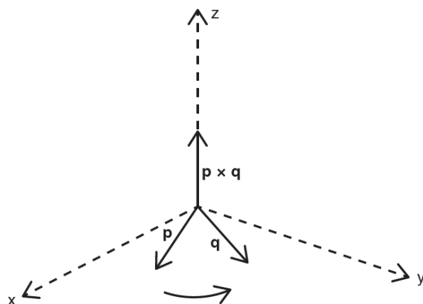
图 4.2: 叉积的右手定则。如果你把右手的手指顺着从 p 到 q 的箭头所示方向弯曲——在本例中是逆时针方向——你就能从拇指的方向得到 p \times q 的方向：它将指向朝上、即 z 的正方向。要找出 q \times p 的方向，你必须把右手翻转过来，让手指顺时针弯曲，此时你的拇指将朝下，指向 z 的负方向。本例中 p 与 q 都在 x - y （水平）平面内，但无论它们位于哪个平面，它们的向量积都会垂直于该平面。
