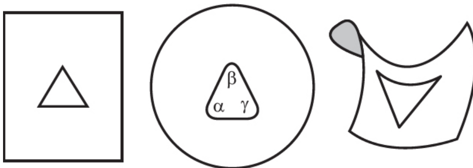
图 10.4: 在一张平纸上，三角形中的角 \alpha, \beta, \gamma 之和为 180^\circ (即 \pi 弧度)；但在球面上，它们的和大于 \pi ；而在马鞍面上，它们的和小于 \pi 。
