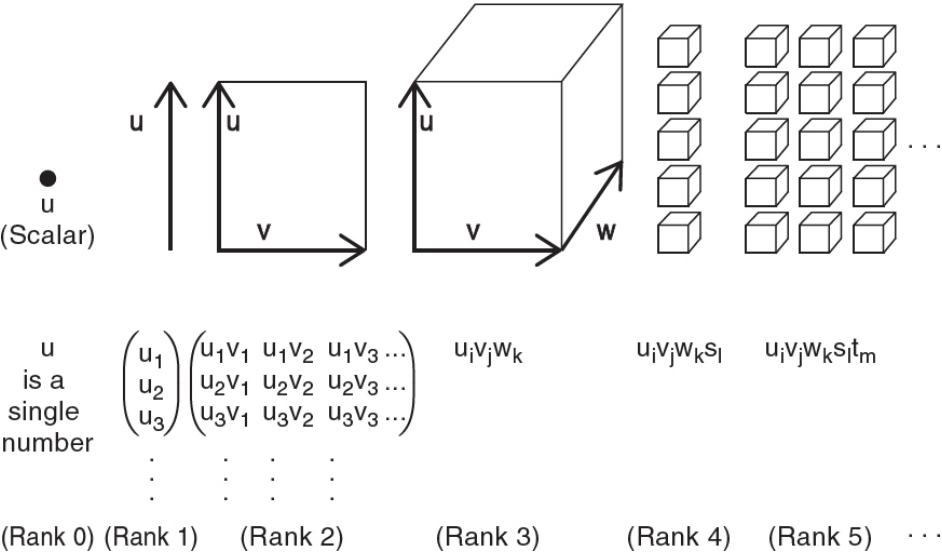
图 11.1: 张量（或外）积把参与相乘的那些张量的信息合并起来。普通的数用诸如 a 这样的符号来表示。如果它们表示的是不依赖于坐标的量——比如温度——那么它们就是标量，而既然标量在坐标变换下不变，它们就是张量。我们会看到向量也是张量，而我们此前也已经看到，它们的分量用一个指标来标记，这个指标代表测量该分量所沿的那条轴。列向量 \mathbf{u} 与行向量 \mathbf{v} 的张量积 (tensor product) 可以表示成一个矩阵。你可能熟悉用符号 a_{ij} 表示矩阵第 i 行第 j 列的元素，所以这里 a_{ij} = u_i v_j 。我会在正文的二维例子中详细说明这一点。同样地，你可以构造出更多的张量积。例如，单指标向量 \mathbf{u} 与矩阵 A 的张量积，其分量带有 3 个指标，你在正文中也能看到。类似地，如果矩阵 A 与 B 各自都由向量的外积构成，那么它们的张量积的分量就是 c_{ijkl} \equiv u_i v_j w_k s_l ，如此等等。这并不是构造新张量的唯一方式，但请注意，随着张量的“秩 (rank)”增大，你能表示的信息就更多。这个“秩”也叫张量的“阶 (order)”，因为里奇提出这个想法时就是这么称呼它的。它与从一个坐标系变换到另一个坐标系所需要的变换矩阵的个数有关，但本质上它对应于指标的个数，每一个指标代表着一种不同类型的信息。（如果你熟悉矩阵代数，请注意：对于被视为张量的矩阵而言，这里“秩”的用法与线性代数中的用法不同。）关于这一点，我们后面还会看到更多。
