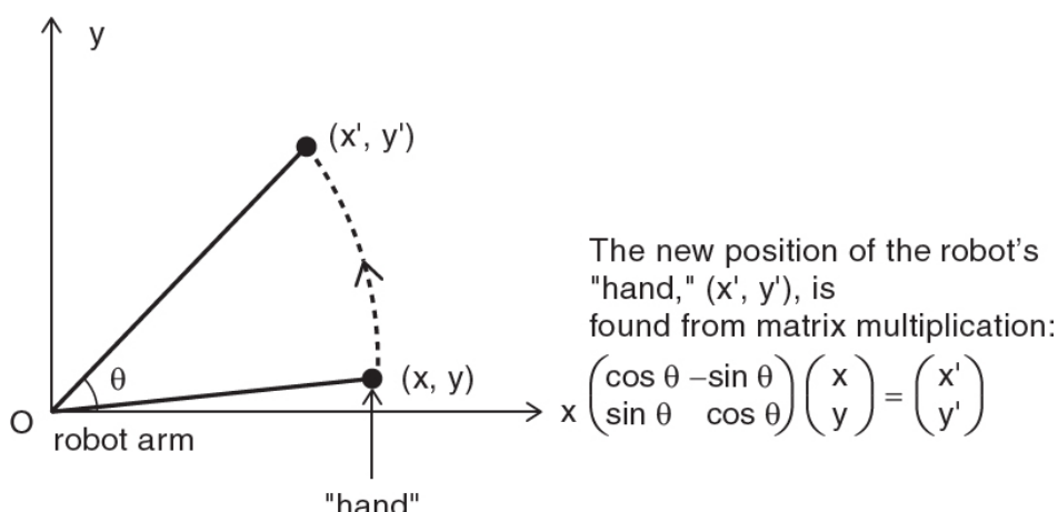
图 4.3: 绕 x - y 平面的原点、用旋转矩阵把一条机械臂逆时针转过角 \theta 。当你把这个矩阵方程的左端乘开，所得的那组方程——它说明如何用 x 和 y 写出 x' 与 y' ——就代表一个线性变换。不过这里的细节并不那么重要：关键是变换方程这个想法。
