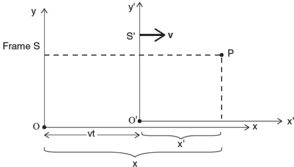
图 9.5: 两个参照系 S 与 S' 以这样的方式相对运动: S' 相对于 S 以恒定速度 v 向右运动。所以, 我们不妨把 S 当作站在人行道上的你, 把 S' 当作开车经过的某个人。如果两根轴起初是重合的——如果在时刻 t = 0 你与那辆车彼此齐平——那么经过一段时间 t 之后, S' 参照系 (那辆车) 就会向右移动 vt 个单位。在这种情形下相对运动是水平方向的, 所以对于任意一点 P , 它的 y 与 y' 坐标 (在三维中还有 z 与 z' 坐标) 是相同的; 然而在时间 t 这段里, S' 已经移近了 P , 所以在那一时刻所做的一次量度会给出: P 的水平坐标在 S 参照系中量得为 x , 而在相对于运动的 S' 参照系量得为 x' (= x - vt) 。这是牛顿式 / 伽利略式的观点, 其中时间对两位观测者都以同样的速率流逝。即便如此, 你也可以看出, 距离的量度在不同而又相对运动的参照系中必然不同, 因此速度也必须以不同的方式被量度。你可以在相关的 (而且完全可选的!) 知识框里看到这一点在数学上的后果, 既有牛顿式的观点, 也有爱因斯坦式的观点。
