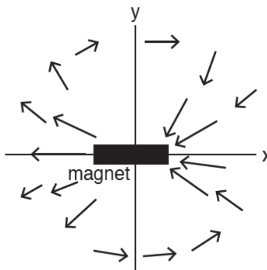
图 6.6: 事后看来, 你可以看到图 6.3a 中那些由铁屑构成的、物理上真实存在的线, 怎样在数学上被表示为一个向量场。箭头指向该点上力的方向, 而它们的长度表示力的强度——所以在靠近磁铁两极、力最强的地方, 箭头更长。
