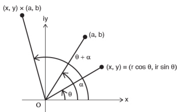
图 3.8: 用旋转表示的复数乘法。
