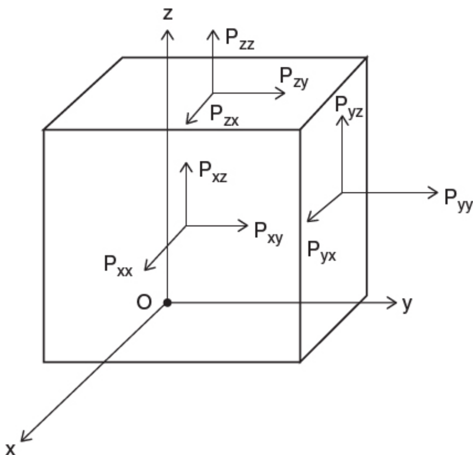
图 9.7: 作用在立方体各个面上的基本应力分量。麦克斯韦指出，如果 P_{hk} = P_{kh} ，这些应力就不会产生转动（他感兴趣的是由磁性产生的转动——正如他的旋度方程所表达的）。确实，这幅图提示：如果比方说 P_{yx} > P_{xy} ，那么右面就会被向前拉，立方体就会开始转动。
