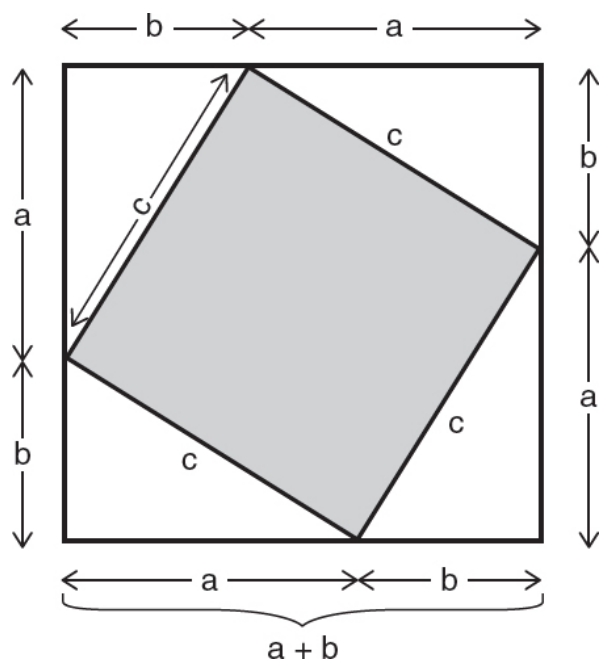
图 1.1 证明毕达哥拉斯定理。所需的直角三角形复制四份，拼成大正方形的四个角。三角形的斜边为 c ，因此你从大正方形（其边长为 a+b ）的面积中减去四个三角形的总面积（即 4 倍的 \frac{ab}{2} ），就得到阴影正方形的面积 c^2 ： c^2 = (a+b)^2 - 4 \cdot \frac{ab}{2} = a^2 + b^2
