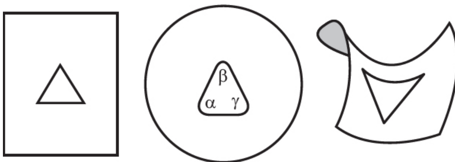
图 10.3 在一张平纸上，三角形中的角 \alpha 、 \beta 、 \gamma 之和为 180^\circ （即 \pi 弧度）；但在球面上，它们的和大于 \pi ；而在马鞍面上，它们的和小于 \pi 。
