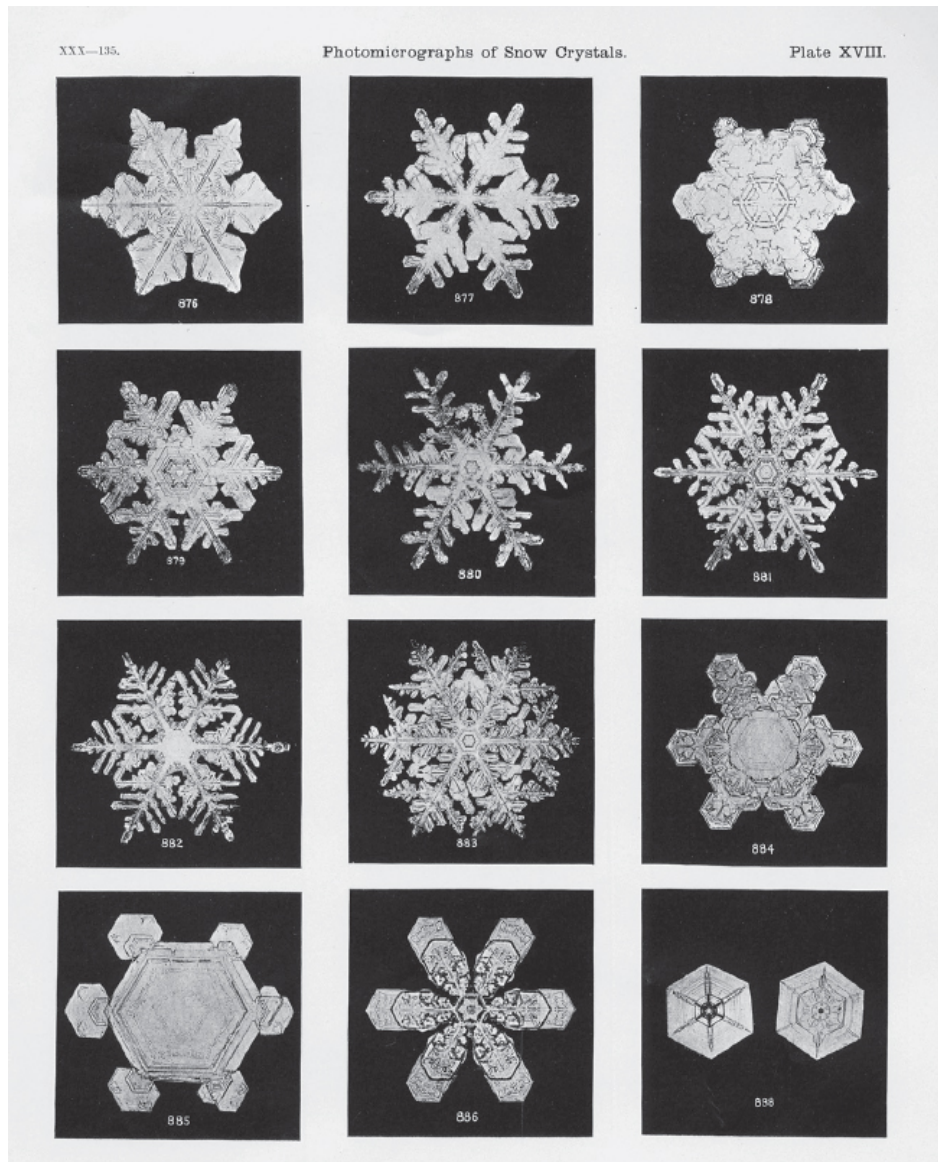
图 9.2 雪花的对称性。图版 18，选自威尔逊·A. 本特利（Wilson A. Bentley）的《1901—1902 年冬季雪晶研究，附前几个冬季所采集的补充数据》（“Studies among the Snow Crystals during the Winter of 1901-2, with Additional Data Collected during Previous Winters”），载 Monthly Weather Review 30，第 13 期（1903 年）：607-16， https://doi.org/10.1175/1520-0493-30.13.607 。
