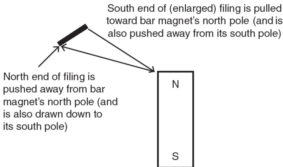
图 6.3B 使每一片铁屑（每一片都像一根小小的条形磁铁）排列起来的那些力。法拉第也对电做了同样的事情：在一个中心电荷周围的空中各处放上一个小小的电“检验”电荷，并留意力在每个位置上如何作用。以这种方式，他构建出了电场与磁场的图景。
