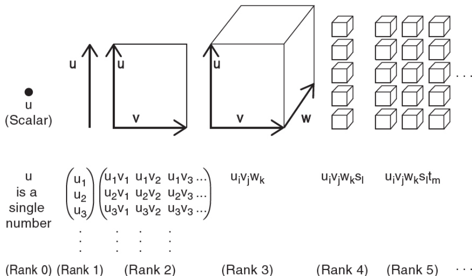
图 11.1 张量（或外）积把参与相乘的那些张量的信息合并起来。普通的数用诸如 a 这样的符号来表示。如果它们表示的是不依赖于坐标的量——比如温度——那么它们就是标量，而既然标量在坐标变换下不变，它们就是张量。我们会看到向量也是张量，而我们此前也已经看到，它们的分量用一个指标来标记，这个指标代表测量该分量所沿的那条轴。列向量 u 与行向量 v 的张量积 (tensor product) 可以表示成一个矩阵。你可能熟悉用符号 a_{ij} 表示矩阵第 i 行第 j 列的元素，所以这里 a_{ij} = u_i v_j 。我会在正文的二维例子中详细说明这一点。同样地，你可以构造出更多的张量积。例如，单指标向量 u 与矩阵 A 的张量积，其分量带有 3 个指标，你在正文中也能看到。类似地，如果矩阵 A 与 B 各自都由向量的外积构成，那么它们的张量积的分量就是 c_{ijkl} \equiv u_i v_j w_k s_l ，如此等等。这并不是构造新张量的唯一方式，但请注意，随着张量的“秩 (rank)”增大，你能表示的信息就更多。这个“秩”也叫张量的“阶 (order)”，因为里奇提出这个想法时就是这么称呼它的。它与从一个坐标系变换到另一个坐标系所需要的变换矩阵的个数有关，但本质上它对应于指标的个数，每一个指标代表着一种不同类型的信息。（如果你熟悉矩阵代数，请注意：对于被视为张量的矩阵而言，这里“秩”的用法与线性代数中的用法不同。）关于这一点，我们后面还会看到更多。
