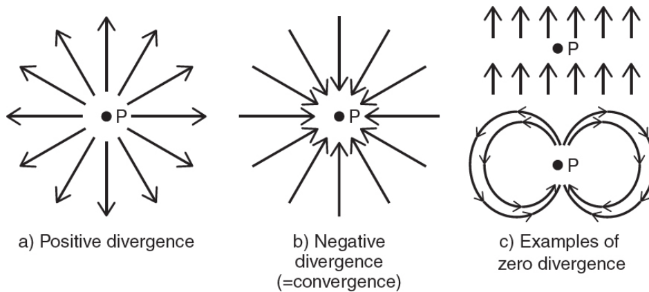
图 7.1 散度。举个例子，库仑定律告诉我们：如果在 P 处有一个带正电的粒子，而你吧单位正试探电荷放在 P 周围场中的不同位置上，那么电力的方向就如图 (a) 中的箭头所示。随着你远离 P ，力按平方反比定律衰减，所以箭头会变小。如果试探电荷是负的，它会被 P 处的正电荷吸引，于是你就得到了情形 (b)。在《电磁通论》( Treatise on Electricity and Magnetism ) 第 1 卷 (第 77 节) 中，麦克斯韦借助高斯关于库仑定律与通量相关的想法，把这个定律写成 \frac{\partial X}{\partial x} + \frac{\partial Y}{\partial y} + \frac{\partial Z}{\partial z} = 4\pi\rho ，其中方程的左边是电力的散度 (他把它分量写作 X, Y, Z )，而 \rho 是场的电荷密度。我在第 6 章的一条尾注中说明过麦克斯韦是如何利用通量的想法推导出这个方程的。(c) 中下面那幅图看上去像条形磁铁周围的力线，如图 6.3a 所示——而我们后面会看到，麦克斯韦的又一个方程说的是磁场的散度为零。
