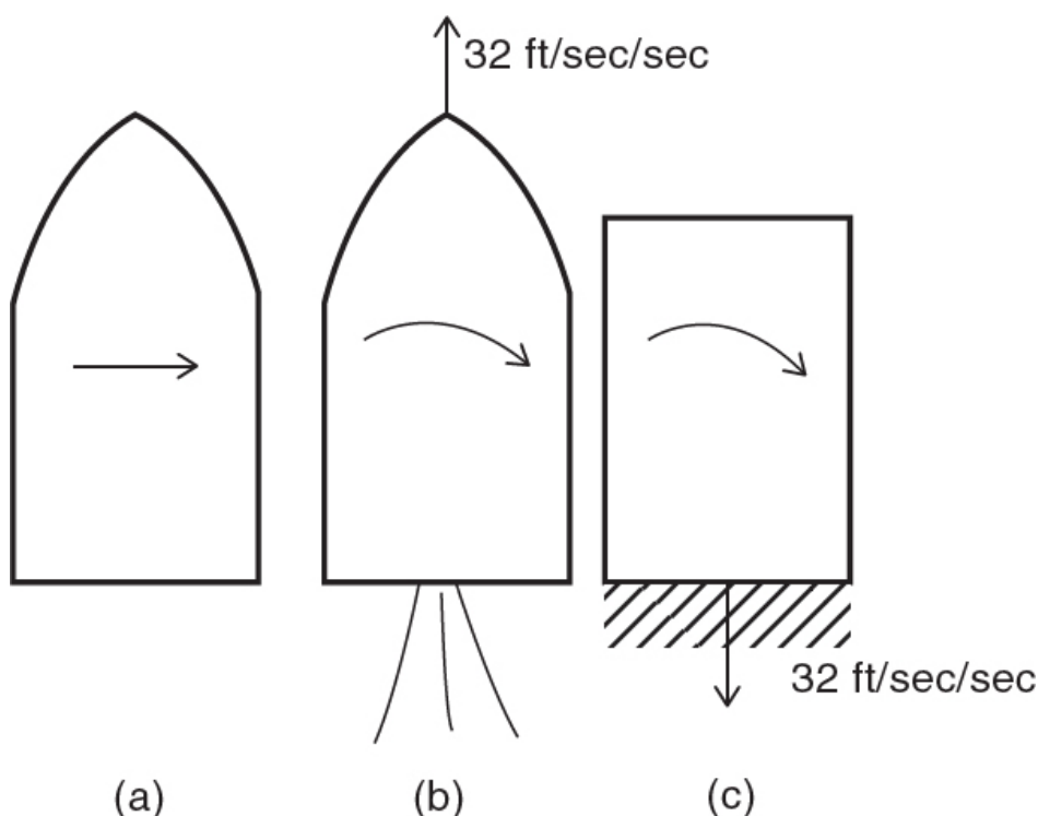
图 12.1: 等效原理。图中显示三个参照系: (a) 一个“惯性”系, 比如一艘无引力(自由漂浮)的宇宙飞船, 或者一个自由下落的人或电梯; (b) 一艘以 32\text{ft/sec/sec} (即 9.8\text{m/sec/sec} ) 向上加速的宇宙飞船或电梯; (c) 地球上这里的一个房间。在 (b) 中, 当宇宙飞船或电梯向上加速时, 它的地板向上推你, 你会感觉与在地球上(参照系 (c)) 一样重——地球也正是在向上推我们, 以回应我们 32\text{ft/sec/sec} 即 9.8\text{m/sec/sec} 的向下引力加速度。(这些数值取自地球表面海平面处的引力加速度; 当然, 在更高的海拔上, 加速度会按牛顿的平方反比定律减小。)在惯性系 (a) 中, 在没有力的情况下, 抛射体一旦被抛出就会以恒定的速率沿直线运动。这就是牛顿第一定律——惯性定律, “惯性系”一词正由此而来。在 (c) 中, 抛射体走一条向下的抛物线路径, 正如哈里奥特和伽利略所表明的那样——而在 (b) 中发生的情形相同, 因为 (b) 与 (c) 是等效的。(随着宇宙飞船向上加速, 地板迎着抛射体升上来, 所以外部的观测者会看到抛射体越来越靠近地板。换句话说, 它的路径看上去是弯的。)类似地, 一道从火箭或电梯的一侧射向另一侧的光线, 在参照系 (a) 中是直的, 但在 (b) 中地板会升上去迎接它, 于是对外部观测者来说它看上去是弯的。既然 (b) 与 (c) 等效, 爱因斯坦便推导出: 引力会使光线弯曲。
