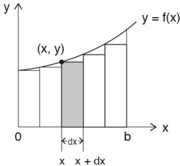
图 2.1: 曲线下的面积。带阴影的矩形对应于图上一般的点 (x, y) ，它的面积 (长乘宽) 是 ydx 。当你对函数 y = f(x) 在 x = 0 与 x = b 之间“积分”时，你实际上是在求 dx 为无穷小时所有这些矩形的和。这个积分写作 \int_0^b ydx ，更具体地说，对于这个函数，是 \int_0^b f(x) dx ，它等于 x 轴与曲线 f(x) 之间、 x 取值在 0 与 b 之间的那块面积。
