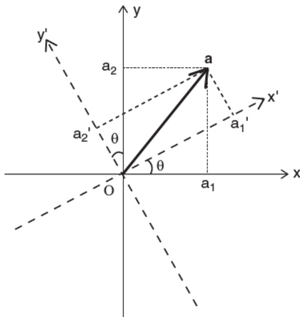
图 9.1: 向量 \mathbf{a} 在通常的 x - y 参照系中具有分量 (a_1, a_2) ，而在旋转后的 x' - y' 参照系中具有 (a_1', a_2') 。它是同一个向量，却有两种不同的坐标表示。正如你从图中的几何所看到的，向量的长度在两个参照系中是相同的。用数学的语言说，它在旋转下是不变的。对第二个向量 \mathbf{b} 也同样成立。所以数量积与向量积在旋转下也是不变的，你利用这些积的几何定义就可以看出： \mathbf{a} \cdot \mathbf{b} = ab \cos \Phi ，其中 a 和 b 是两个向量的长度， \Phi 是它们之间的夹角；因为向量本身没有改变，它们之间的夹角就不受坐标改变的影响。类似地， \mathbf{a} \times \mathbf{b} 的模（长度）是 ab \sin \Phi ，方向垂直于这两个向量所在的平面，而这个平面——在这里的图示中就是纸面——当你以这种方式旋转坐标轴时并不改变。当坐标轴像这样被改变时，“坐标变换方程”是： x' = x \cos \theta + y \sin \theta ， y' = -x \sin \theta + y \cos \theta 。我们在图 4.2 中看到过这种做法的一个例子（在那里我们旋转的是机械臂，而不是坐标轴）。但关键的并不是细节，而是这样一个事实：当你改变你的坐标参照系时，两组坐标是由特定的方程联系起来的。这是张量这一想法的关键。
