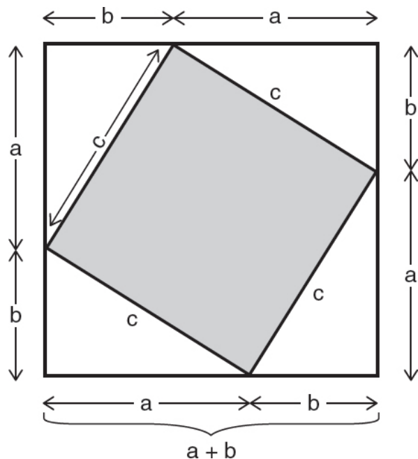
图 1.1: 证明毕达哥拉斯定理。所需的直角三角形复制四份, 拼成大正方形的四个角。三角形的斜边为 c , 因此你只消从大正方形 (其边长为 a+b ) 的面积中减去四个三角形的总面积 (即 4 倍的 \frac{ab}{2} ), 就得到阴影正方形的面积 c^2 : c^2 = (a+b)^2 - \frac{4ab}{2} = a^2 + b^2
