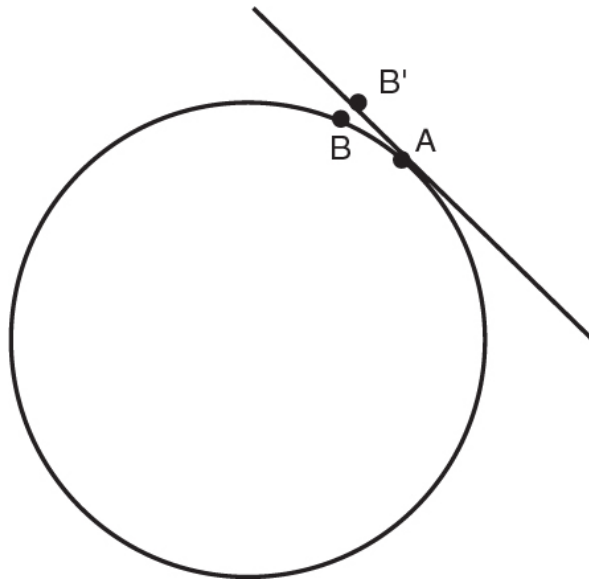
图 10.2: 当一条曲线、或者一个曲面上的两点靠得非常近时，它们之间的距离 AB 近似等于直线距离 AB' 。例如在计算机图形学中，曲线就可以由一段段极小的切线段拼接而成。
