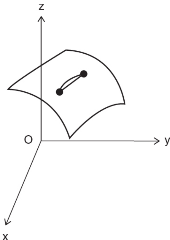
图 10.3: 两点之间相隔无穷小距离时, 它们之间的弯曲距离几乎就等于在 3 维空间中量出的、仿佛曲面并不存在时的直线距离。
